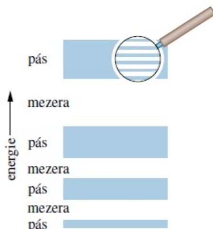
Obrázek 1: Pásová struktura pevné látky. Zvětšený pohled ukazuje, že každý pás se skládá z velmi velkého počtu velmi blízkých energetických hladin.
