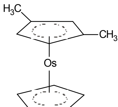
1,3-dimethyl-osmiumocen
