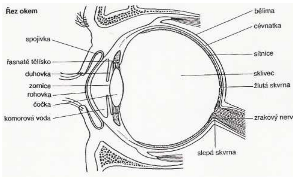
Obr. 12.7.1. Řez okem (převzato: http://fyzika.gbn.cz/phprs/image/fyzika/optika/ )
