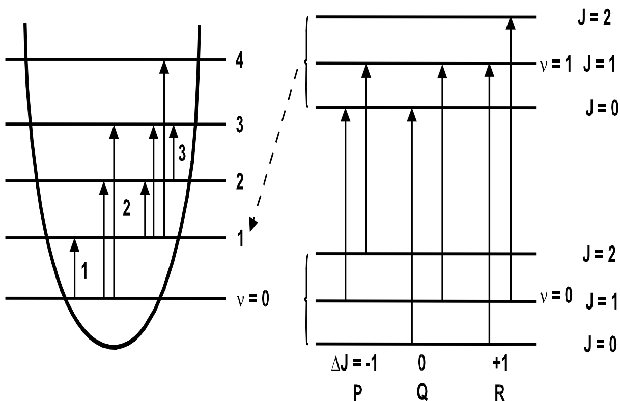
Obr.2. Vibrační (vlevo) a rotační (vpravo) přechody 1-normální, 2-vyšší harmonické, 3-"horké" přechody v -vibrační kvantové číslo, J -rotační kvantové číslo, P,Q,R-větve rotačně vibračního pásu
