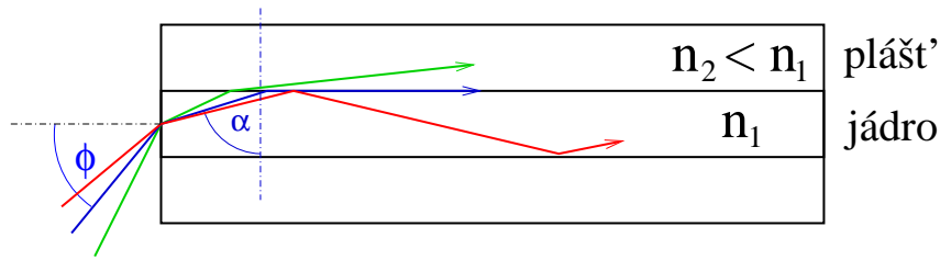
Obrázek 17: Trajektorie meridiánových paprsků v SI vlákně. Zeleně označený paprsek se na rozhraní jádra a pláště láme a je rychle vyzářen ven z vlákna, červeně označený paprsek se totálně odráží a je vláknem veden. \sin \phi se nazývá numerická apertura vlákna.
