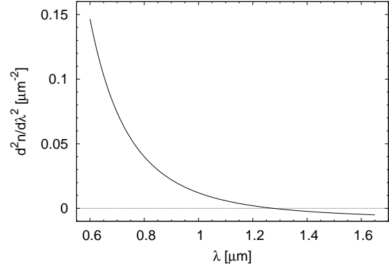
Obrázek 24: Druhá derivace závislosti n(\lambda) křemenného skla.
