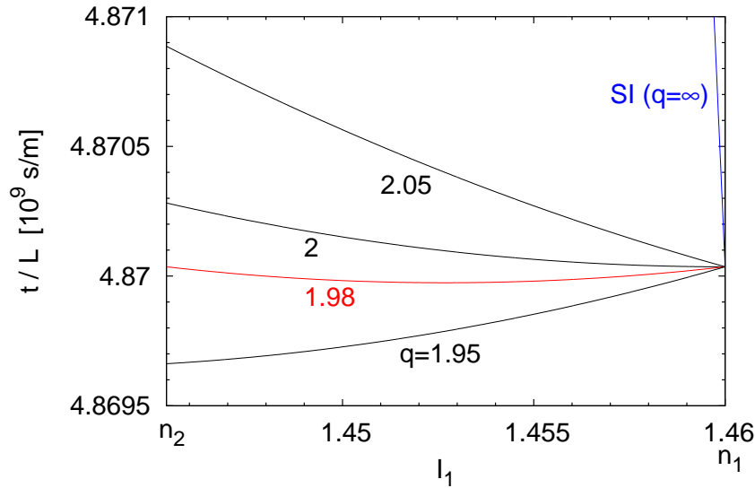
Obrázek 22: Převrácená hodnota grupové rychlosti paprsků spočítaná podle (65) pro několik hodnot parametru q ve vlákne s n_1 = 1,46 a \Delta_n = 0,01 . Červená křivka ( q = 1,98 ) odpovídá ideálnímu profilu podle (67), modrá křivka SI vláknu. Všechny křivky se pro I_1 = n_1 sbíhají v hodnotě n_1/c .
