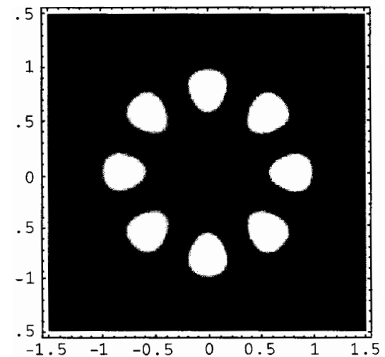
Obrázek 15: Mód LP_{41} . Obr. 10 – 15 byly
