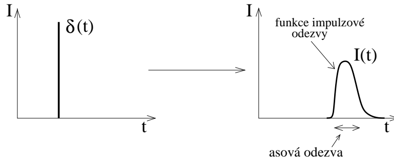
Obrázek 26: Funkce impulzové odezvy je časový průběh intenzity světla na výstupu vlákna, do kterého vstoupil pulz ve tvaru delta funkce.
