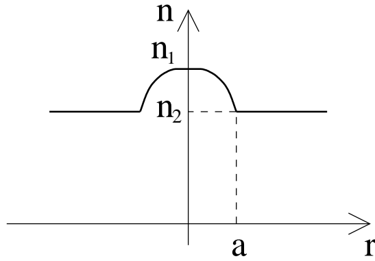
Obrázek 1: Příklad profilu indexu lomu optického vlákna.
