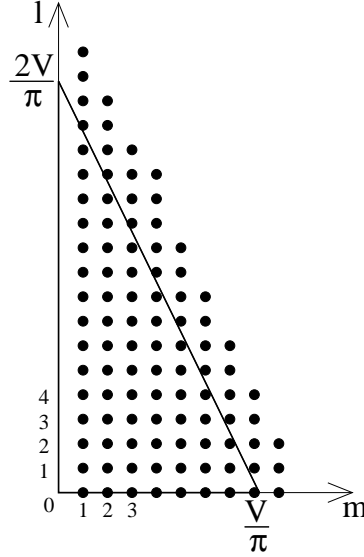
Obrázek 16: Vedené módy splňují podmínku V \geq l\pi/2 + m\pi a leží proto uvnitř plochy znázorněného trojúhelníku. Každému bodu odpovídají čtyři módy lišící se polarizací a znaménkem l .
