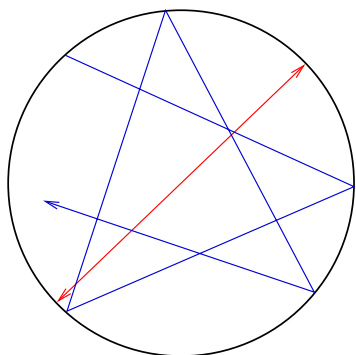
Obrázek 18: Průmět trajektorie meridiánového (červeně) a kosého (modře) paprsku v SI vlákně do roviny xy . Černý kruh označuje hranici jádra a pláště.
