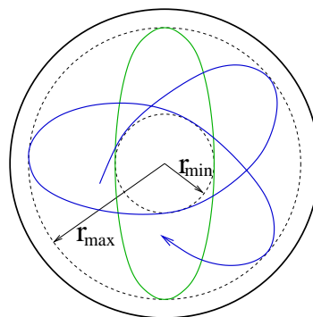
Obrázek 19: Průmět trajektorie kosých paprsků v obecném gradientním (modrá křivka) a parabolickém (zelená elipsa) vlákně do roviny xy .
