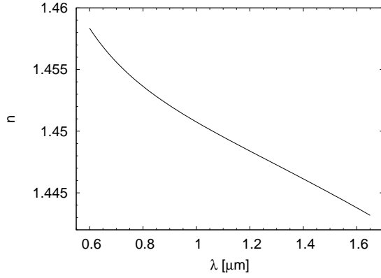
Obrázek 23: Index lomu křemenného skla v závislosti na vlnové délce.
