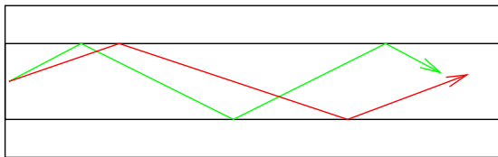
Obrázek 20: Trajektorie paprsků v SI vlákně. Zeleně označený paprsek musí překonat delší dráhu než červeně označený paprsek.
