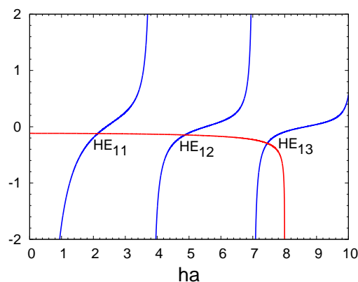
Obrázek 6: Grafické řešení rovnice (35) pro l = 1 . Zvolená podmínka V = 8 vede ke třem HE_1 módům. Podstatná je skutečnost, že průsečík odpovídající módu HE_{11} existuje pro libovolnou hodnotu V .
