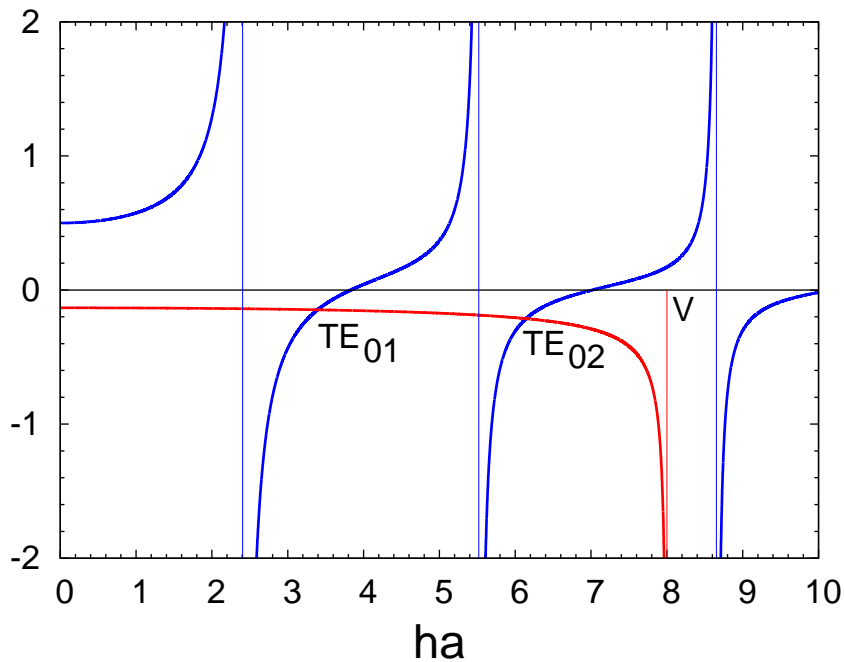
Obrázek 4: Levá (kreslená modře) a pravá (červeně) strana rovnice (31) pro V = 8 .
