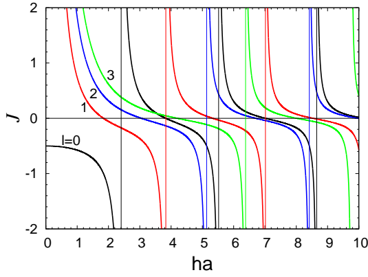
Obrázek 2: Výraz (27) pro řády l = 0 - 3 . Tenkými svíslými čarami jsou znázorněny asymptoty v místech, kde výraz (27) diverguje.
