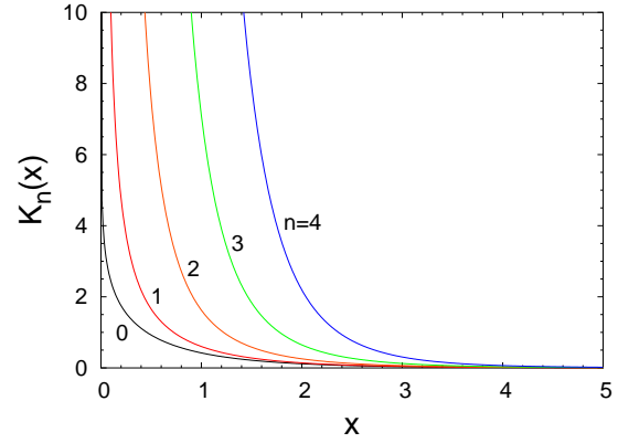
Obrázek 31: Modifikované Besselovy funkce druhého druhu celočíselných řádů 0 až 4.
