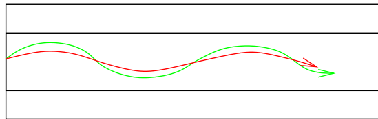
Obrázek 21: Trajektorie paprsků v gradientním vlákně. Zeleně označený paprsek se pohybuje v prostředí s nižším indexem lomu.
