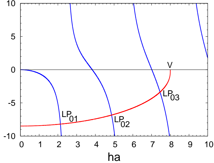
Obrázek 9: Levá (kreslená modře) a pravá (červeně) strana rovnice (42) pro l = 0 a V = 8 .
