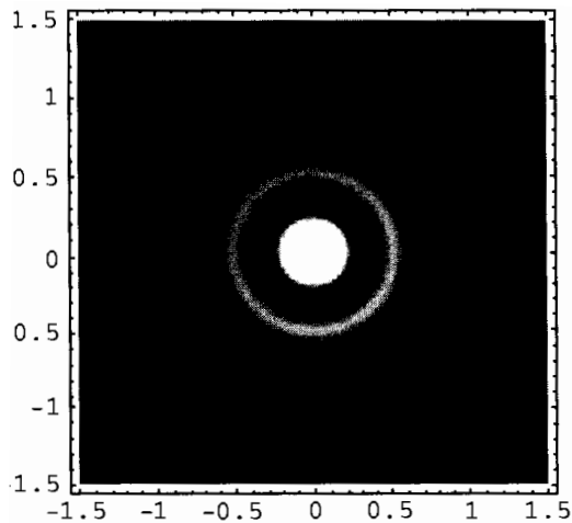
Obrázek 11: Rozložení intenzity světla v optickém vlákně odpovídající modu LP_{03} . Špatný obrázek!!!
