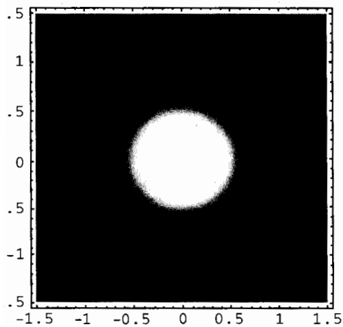
Obrázek 10: Rozložení intenzity světla v optickém vlákně odpovídající modu LP_{01} .
