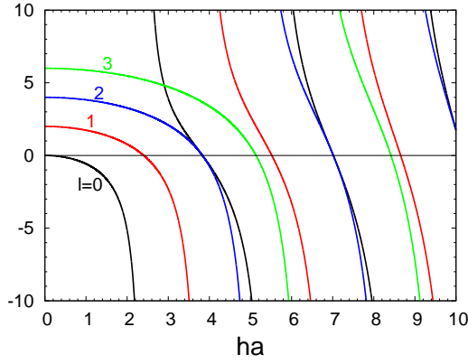
Obrázek 7: Levá strana rovnice (42) pro řády l = 0 (černě), 1 (červeně), 2 (modře) a 3 (zeleně).
