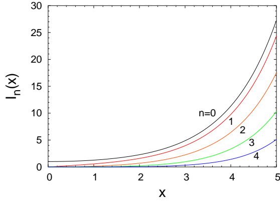
Obrázek 30: Modifikované Besselovy funkce prvního druhu celočíselných řádů 0 až 4.
