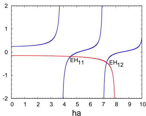
Obrázek 5: Grafické řešení rovnice (34) pro l = 1 a V = 8 . Za zvolených podmínek se levá (kreslená modře) a pravá (kreslená červeně) strana rovnice protínají ve dvou bodech odpovídajících dvěma EH_1 módům.
