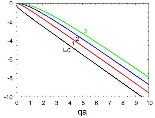
Obrázek 8: Pravá strana rovnice (42) pro řády l = 0 - 3 .
