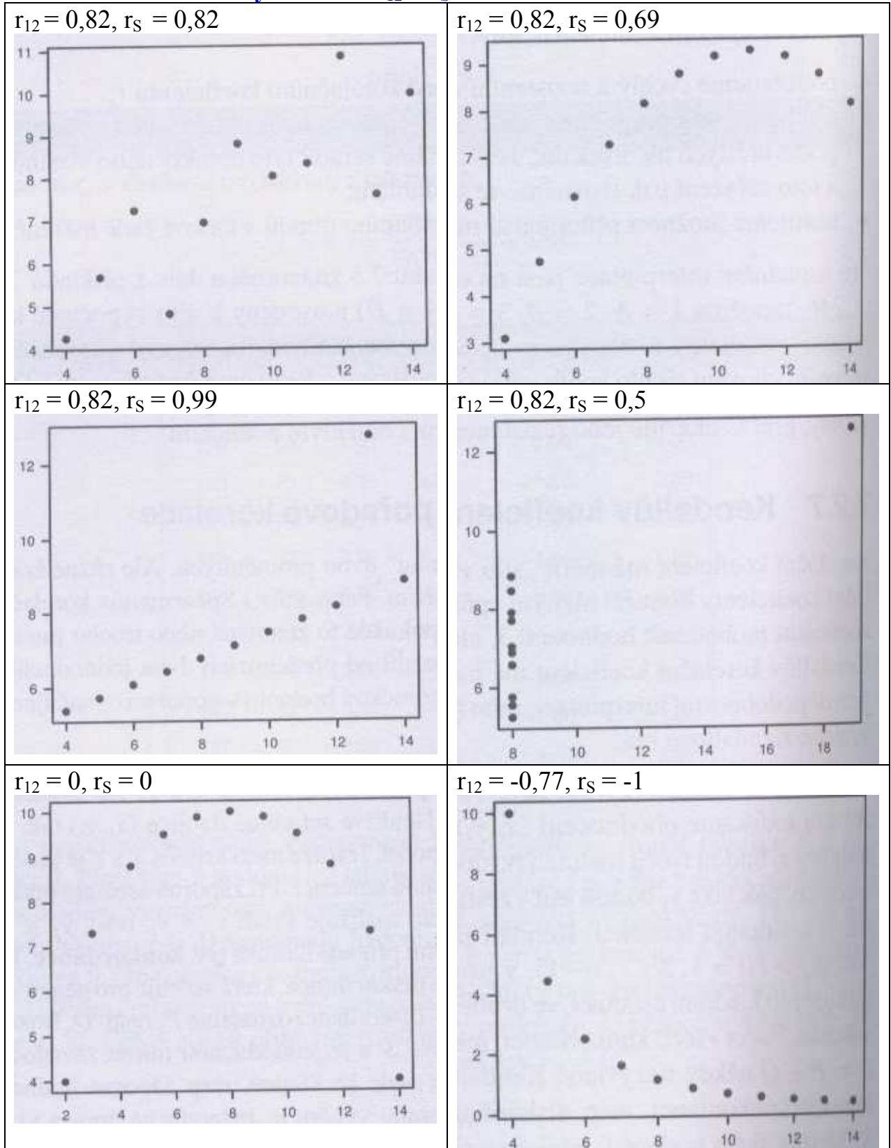
3. obrázek ukazuje odolnost Spearmanova koeficientu vůči odlehlým hodnotám.
