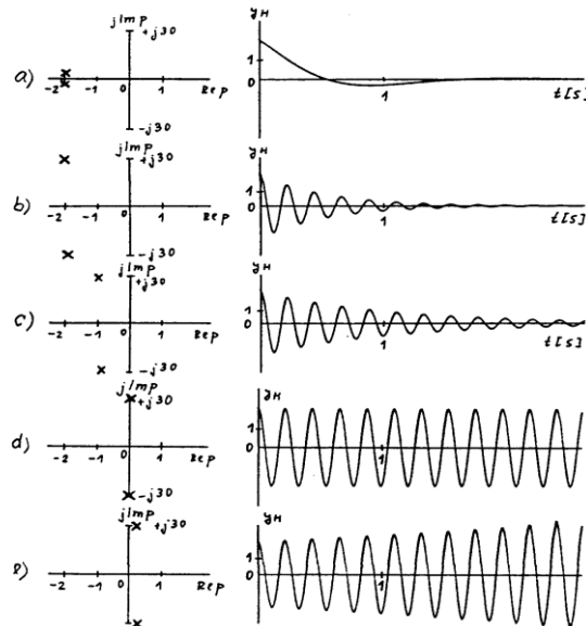
Přirozená odezva systému 2. řádu pro různá rozložení komplexních pólů a integrační konstanty C_1 = C_2 = 1 . a) \lambda_1 = -2 + j3, \lambda_2 = -2 - j3 y_H(t) = 2e^{-2t} \cos(3t) b) \lambda_1 = -2 + j30, \lambda_2 = -2 - j30 y_H(t) = 2e^{-2t} \cos(30t) c) \lambda_1 = -1 + j30, \lambda_2 = -1 - j30 y_H(t) = 2e^{-t} \cos(30t) d) \lambda_1 = j30, \lambda_2 = -j30 y_H(t) = 2 \cos(30t) e) \lambda_1 = 0.2 + j30, \lambda_2 = 0.2 - j30 y_H(t) = 2e^{0.2t} \cos(30t)
