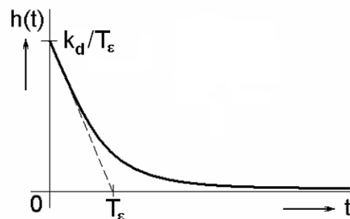
Obr.7-12 Přeběžná charakteristika reálného derivačního članku
