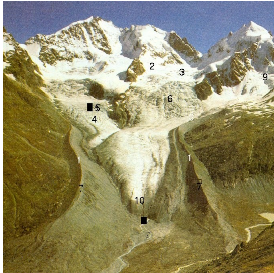
Moraine
