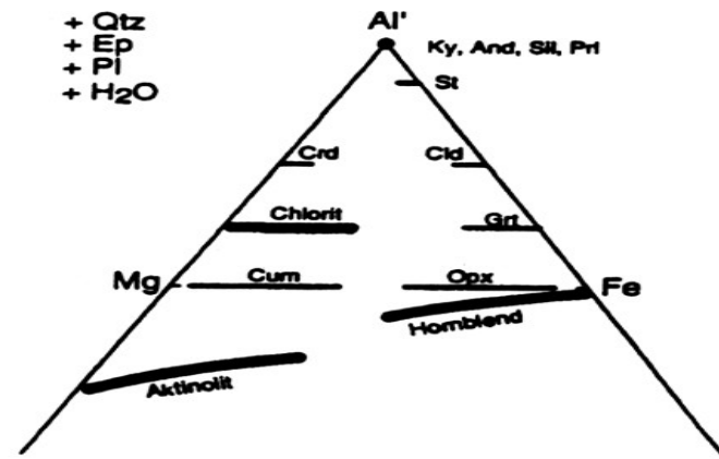
Obr. 5-4. Diagram AFM zobrazený z pozice křemene, epidotu a H 2 O ukazující projekce typických minerálů metabazitů. Převzato ze Speara (1993).
