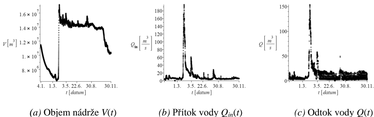
Obr. 8.2 Časové řady objemu nádrže a průtoku vody na přítoku a odtoku.
