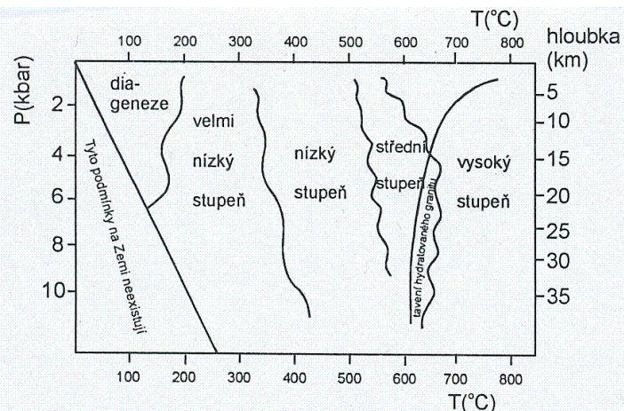
Obr. 1-1. Schematický PT (tlak, teplota) diagram s vyznačením polí pro stupně metamorfózy a diagenézi. V diagramu je také vyznačena křivka tavení hydratovaného granitu a pole podmínek, které na Zemi neexistují.
