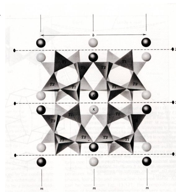
Struktura živce
