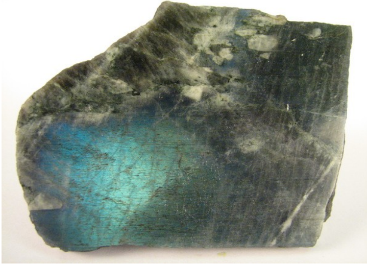
Labradorit
