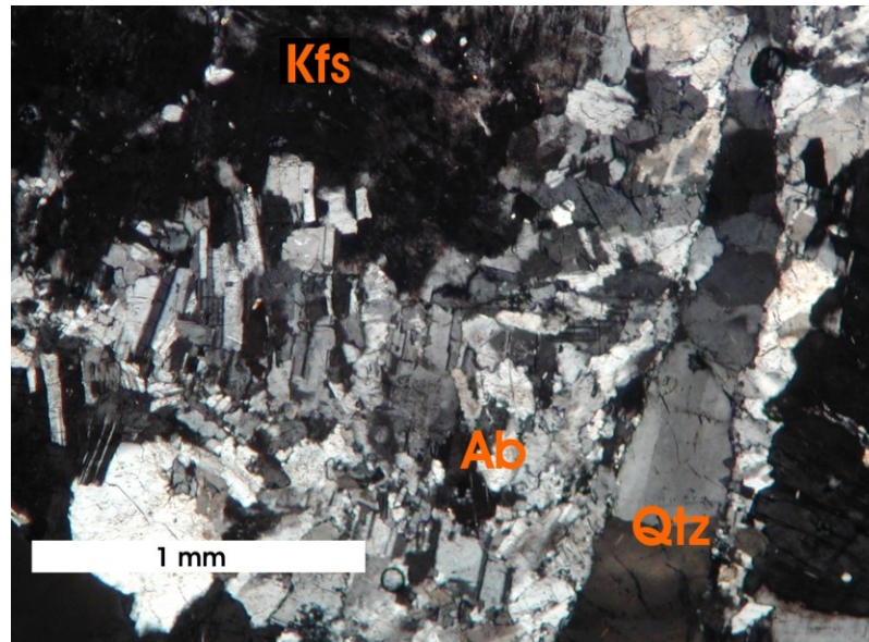
K-živce, Vlastějovice
