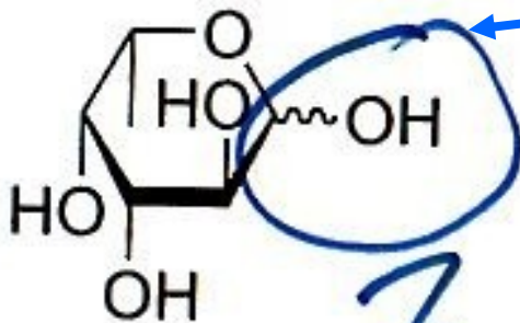
Fukóza
