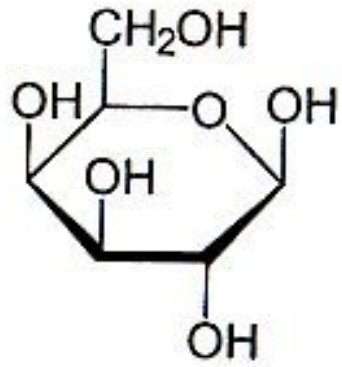
Galaktóza
