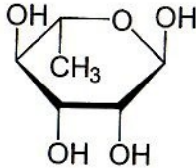
Ramnóza (rhamnose)
