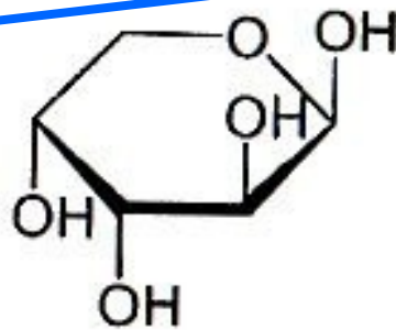
Arabinóza
