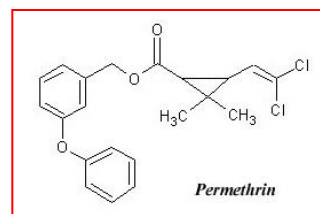
Permethrin
