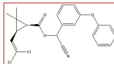
Cypermethrin
