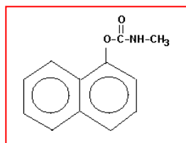
Carbaryl
