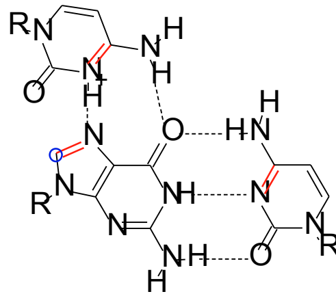
C•G•C + triad (Watson-Crick C•G + Hoogsteen G•C + pairing)
