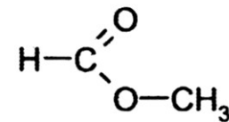
methyl-formiát
