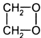
1,2-dioxetan
