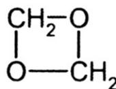
1,3-dioxetan
