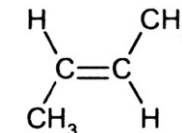
trans-but-2-en
