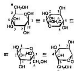
Obr. 8. Různě orientované vzorce \beta -D-glukopyranosy
