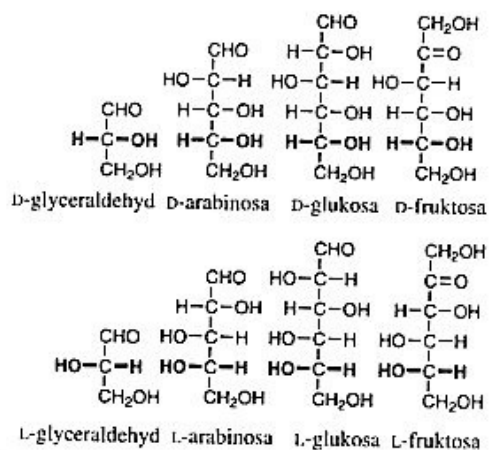
Obr. 3. Příklady Fischerových vzorců některých D- a L-monosacharidů
