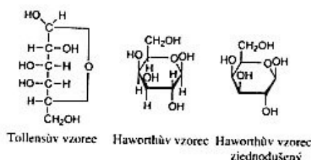
Obr. 6. Tollensovy a Haworthovy vzorce \beta -D-galaktopyranosy
