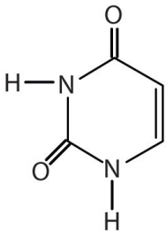
Uracil (U) RNA only
