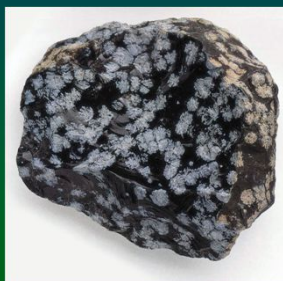
„Vločkový“ obsidián – světlé útvary tvoří sférolity vzniklé při devitrifikaci skla
