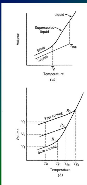
Obr. a: Závislost měrného objemu na teplotě pro krystalickou látku a sklo
