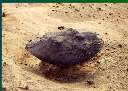
Vulkanická bomba z vulkánu Capelinhos, Azorské ostrovy, zdroj - Wikipedia
