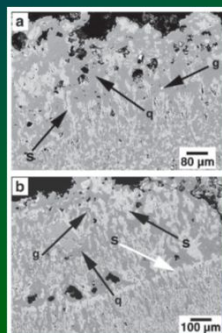
„Vločkový“ obsidián – světlé útvary tvoří sférolity vzniklé při devitrifikaci skla
