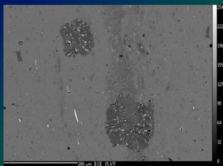
Sférolity v kyselém skle složené z cpx a živců, částečně rozpuštěné ve skle za vzniku „šlírů“.
