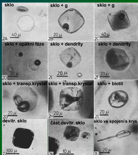
Různé typy inkluzí skla z vyrostlic různých typů vulkanických hornin Japonska (Takenouchi a Imai 1975)
