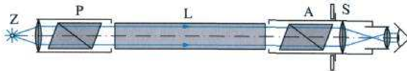
Princip polarimetru
