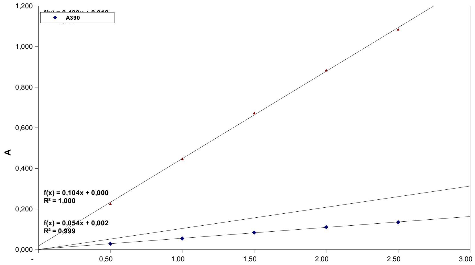
Obr.2. Kalibrační závislosti pro KMnO4
