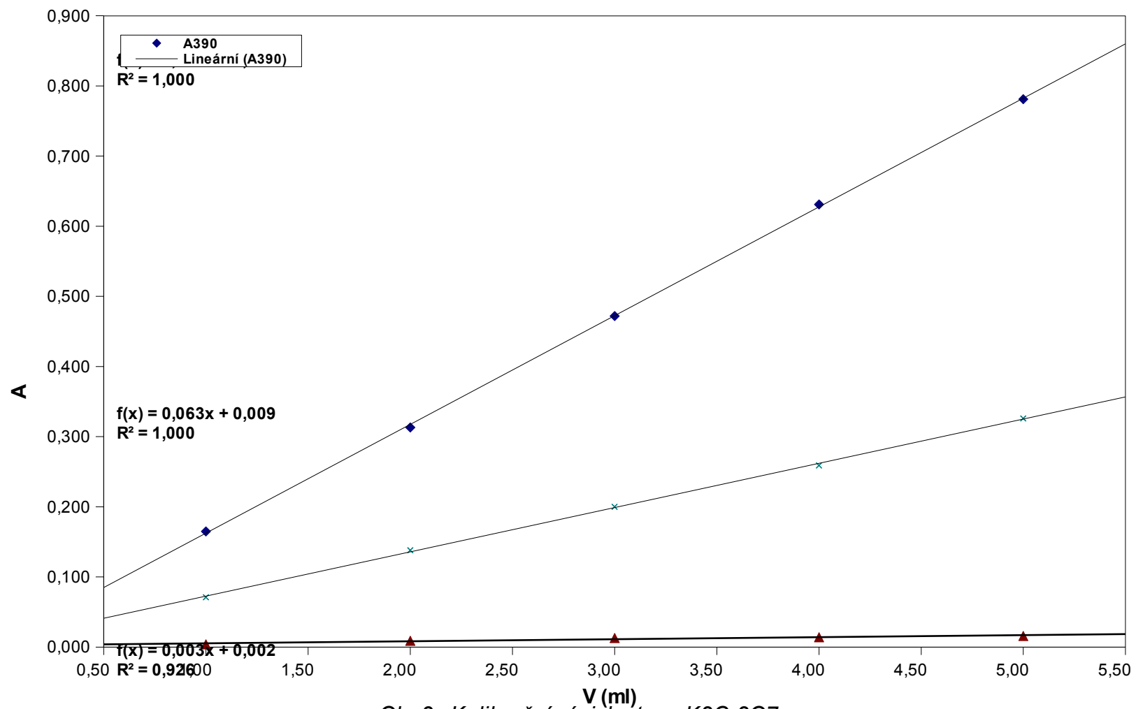
Obr.3. Kalibrační závislost pro K 2 Cr 2 O 7
