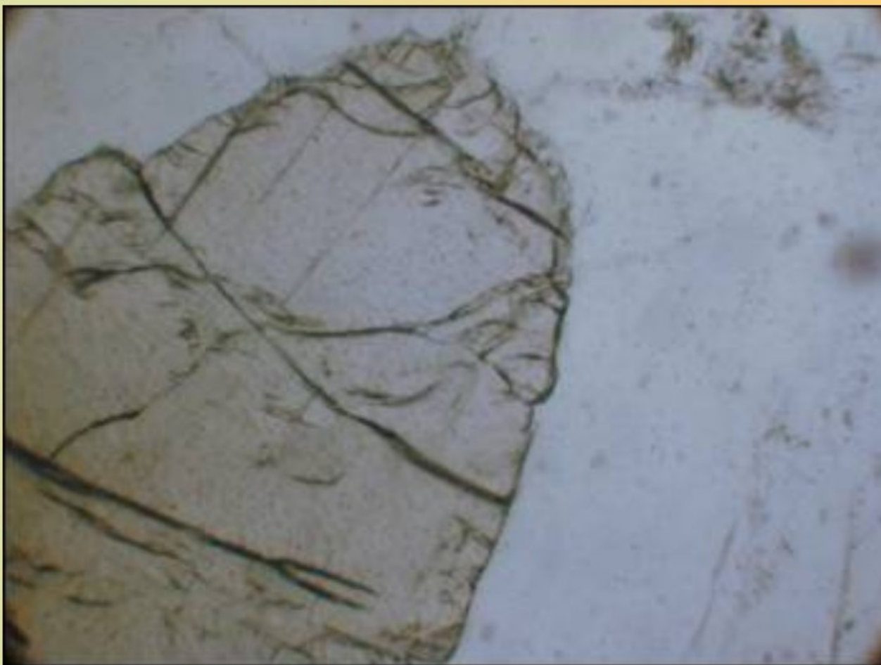
zrno ortopyroxenu v plagioklasu, nápadný je vystupující reliéf, gabro; PPL
