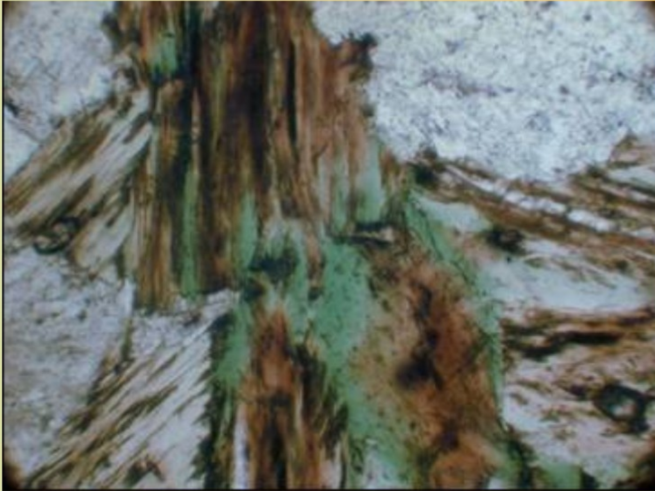
chloritizace biotitu, směr pleochroismu b nebo g, rula; PPL
