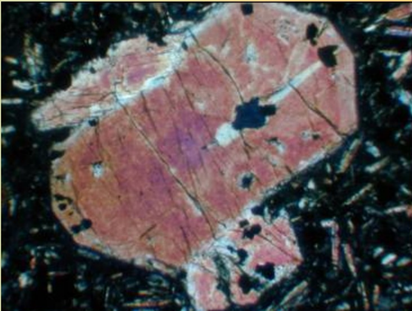
automorfní zrno augitu s charakteristickým dvojlomem; bazalt, XPL
