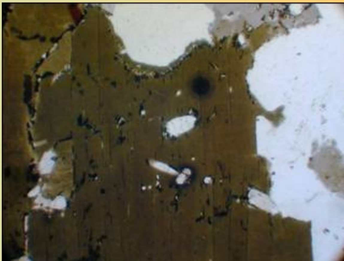
biotit s bazální štěpností, hnědozelené interferenční barvy ve směru b nebo g s inkluzemi zirkonu a apatitu; granit, PPL
