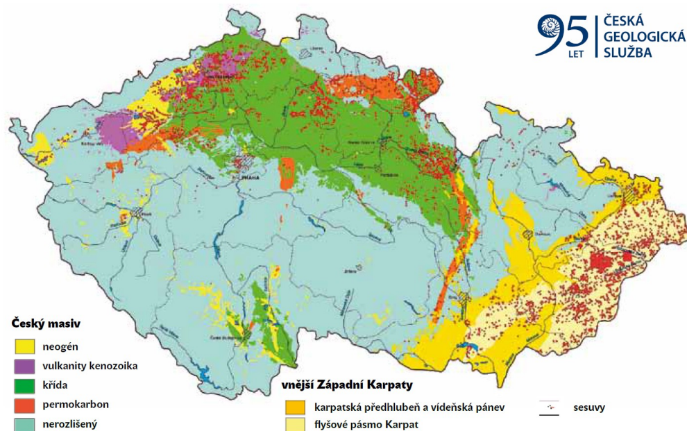
Geologická mapa ČR s vymezením sesuvů podle Krejčí a kol. 2014.
