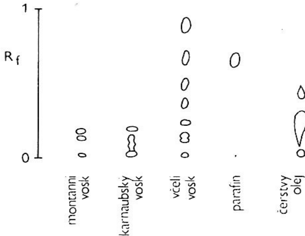
Obr. 22 Tenkovrstvý chromatogram vosků 50 .
