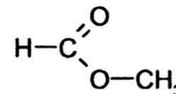
methyl-formiát
