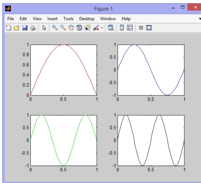
Obr. 9.10: Funkce subplot() .
