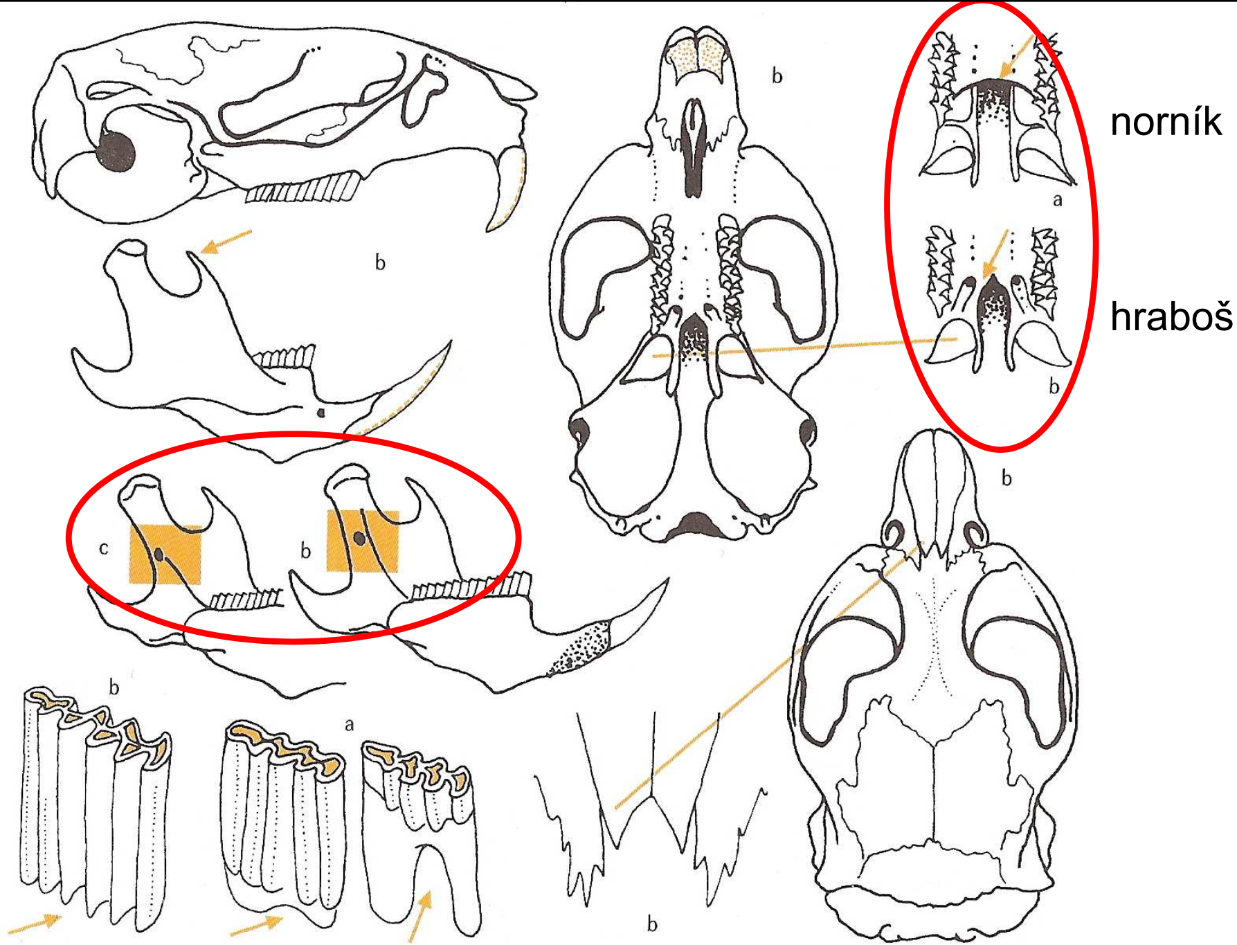
Obr. 118: Lebka hraboše a určovací znaky norníka rudého (a), hraboše polního (b) a h. mokřadního (c)
