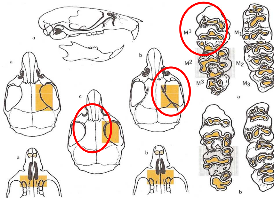
Obr. 126: Lebka a určovací znaky myšice křovinné (i lesní) (a), m. temnopásé (b) a m. malooké (c)
