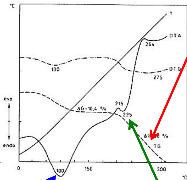
Obr. 12.19. DTA a TG křivky 100 % vlny při ohřeve do 300 °C na vzduchu.
