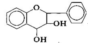
flavan-3,4-ol
