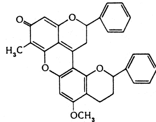
dracorubin
