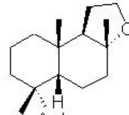
Ambroxan
