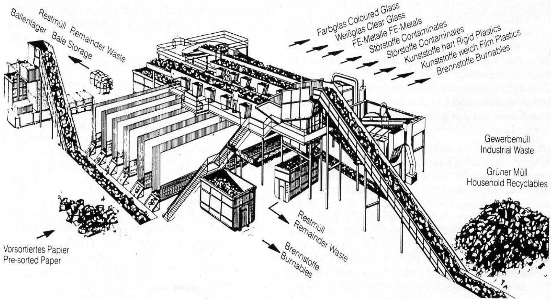
4.10.2021 Bild 5: Sortieranlage für „Grüne Tonne“ und Industrieabfälle
