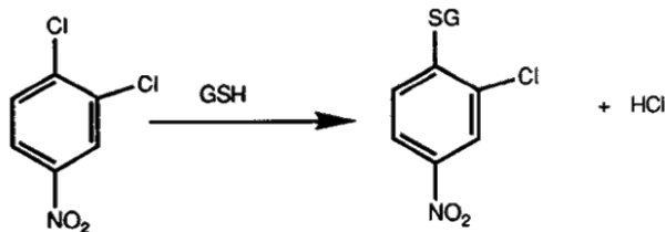
3,4-Dichloronitrobenzene
