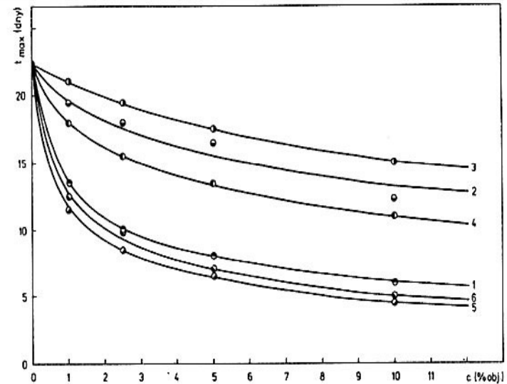
Obr. 18 Doba potřebná k dosažení maxima na křivce tuhnutí lněného oleje v závislosti na koncentraci pigmentu železitá červeně 26 . 1 – anglická červeně, 2 – caput mortuum, 3 – puzo-la, 4 – železitá červeně Lefranc, 5 – Bayferox 130, 6 – červený oxid Winsor Newton.
