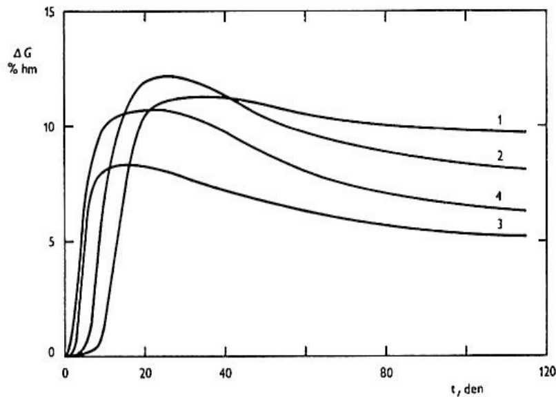
Obr. 17 Závislost přírůstku hmotnosti \Delta G na době stárnutí t při 20 °C filmů lněného oleje s různými pigmenty. 1 – lněný olej bez pigmentu, 2 – lněný olej s blanc fixem, 3 – lněný olej s kobaltovou modří, 4 – lněný olej s anglickou červení.
