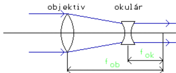
Galileův dalekohled ( 1609 )
