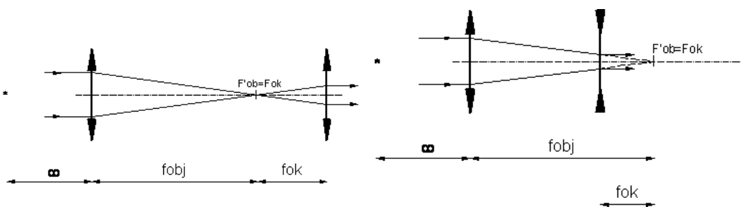
Obrázek 10.7: Schémata Keplerova (vlevo) a Galileova dalekohledu. Autor: Z. Řehoř.
