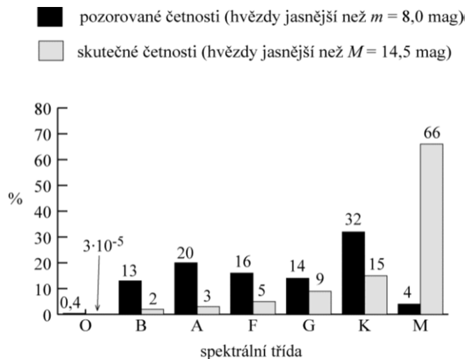
Obrázek 8.9: Četnosti různých spektrálních tříd. Převzato z Pokorný (2006).
