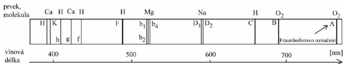
Obrázek 8.2: Fraunhoferovy čáry ve slunečním spektru. Převzato z Pokorný (2006).
