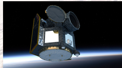
Cheops, start 18. prosince 2019
