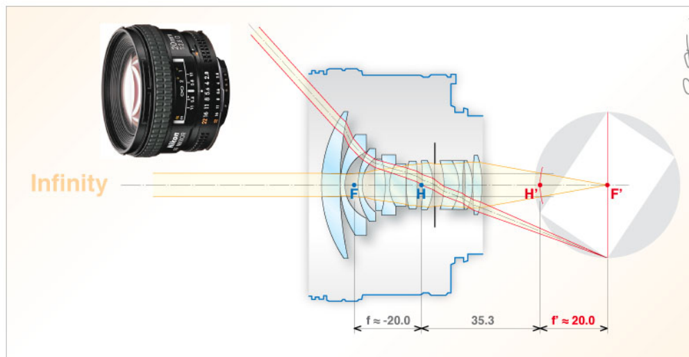
Obrázek 10.11: Efektivní ohnisková vzdálenost je dána vzdáleností H'H' . Převzato z http://www.pierretoscani.com/echo_focal_length.html .
