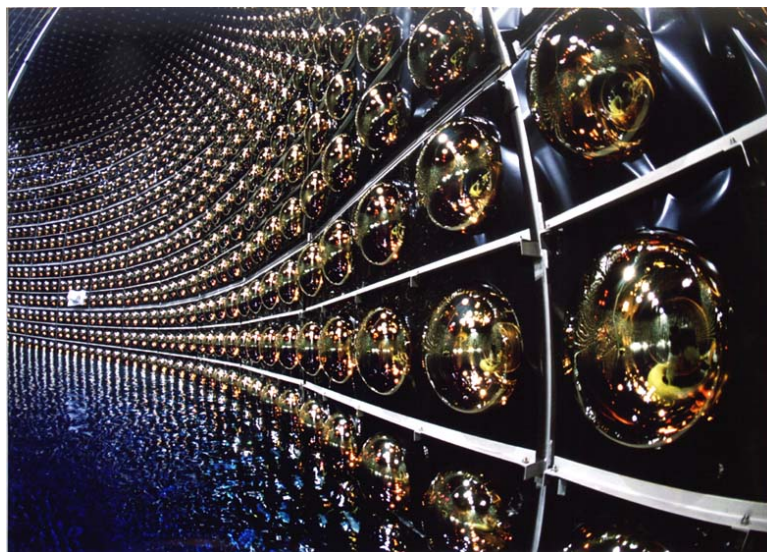
Obrázek 7.8: Skleněné baňky s fotonásobiči v detektoru neutrin Super-Kamiokande. Zdroj: Japan Radio Glass Co.,Ltd.
