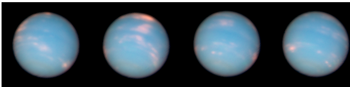
Obrázek 12.22: „Narozeninové“ snímky Neptunu byly pořízeny HST během 16 hodin 25.-26. června 2011. NASA tým připomněla 165 let od objevu planety, za které Neptun dokončil právě jeden oběh kolem Slunce. Zdroj: NASA.
