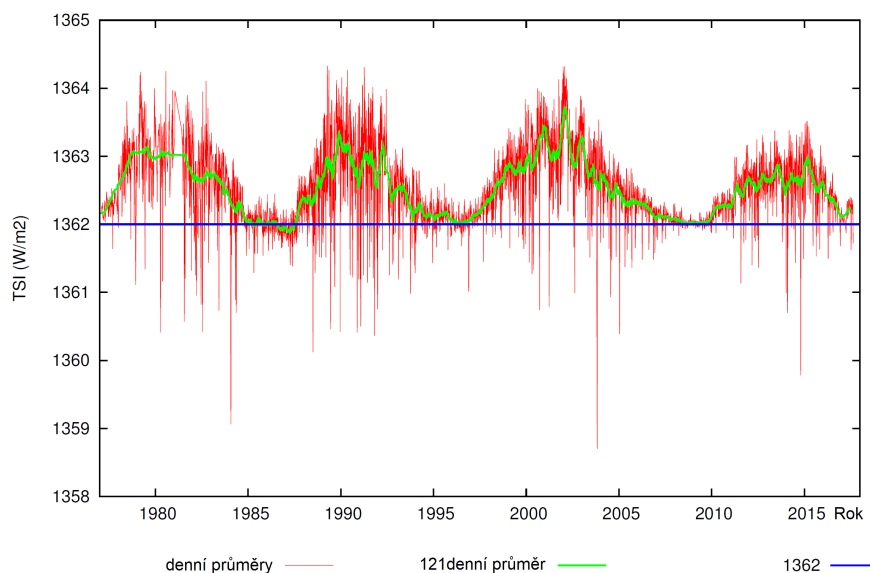
Obrázek 9.1: Měření sluneční konstanty na družicích s využitím různých přístrojů v letech 1979-2017. Změny odpovídají jedenáctiletému cyklu aktivity Slunce (Dewitte & Clerbaux, 2017).
