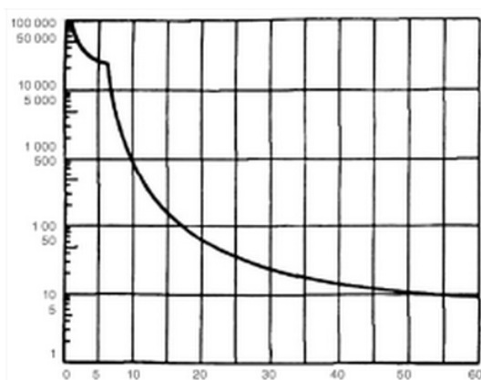
Obrázek 10.3: Typická křivka adaptace na tmou. Na ordinátě (osa y) osvětlení testovací plochy v mikroluxech, na abscise (osa x) trvání adaptace v minutách. Převzato z Boguszaková (2003).
