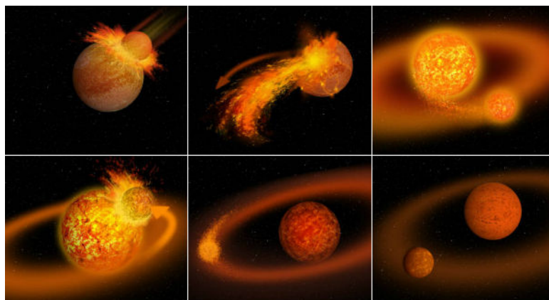
Obrázek 12.26: Simulace vzniku Měsíce při velké srážce s Theiou. Vytvořilo Black Cat Studios.
