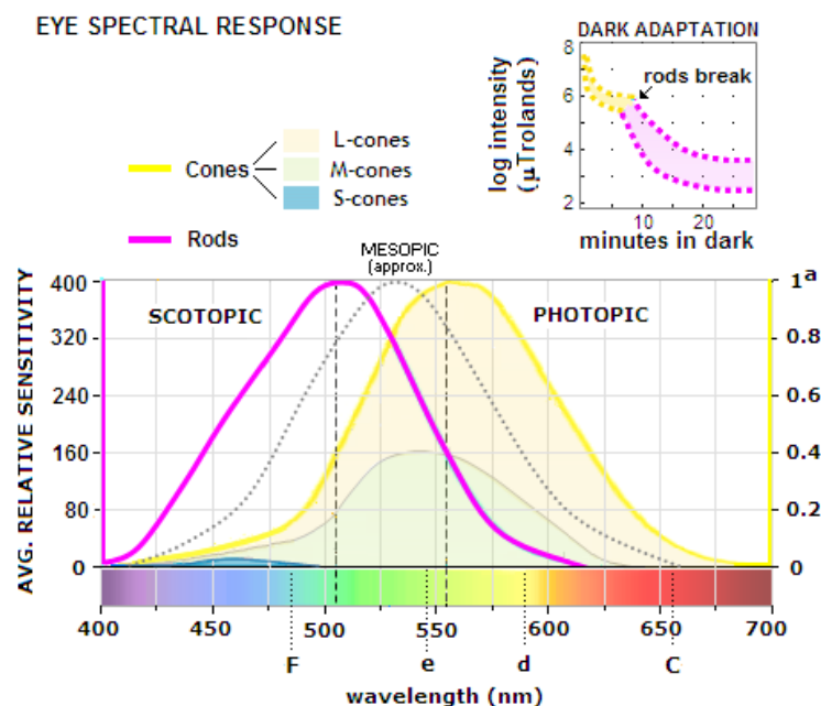
Obrázek 10.2: Spektrální citlivost oka. Vrchol citlivosti čípků je 200krát nižší než vrchol citlivosti tyčinek. Vpravo nahoře: Za špatných světelných podmínek roste citlivost čípků 30krát až 100krát do doby zhruba 10 minut (čím větší je tma, tím rychleji předávají čípky svoji funkci tyčinkám). V okamžiku, kdy se dominantními receptory stanou tyčinky, zvýší se citlivost na 200krát až 1000krát vyšší hodnotu než byl vrchol citlivosti čípků během 20 minut adaptace (citlivosti a doby adaptace jsou velmi individuální). Převzato z http://www.telescope-optics.net .
