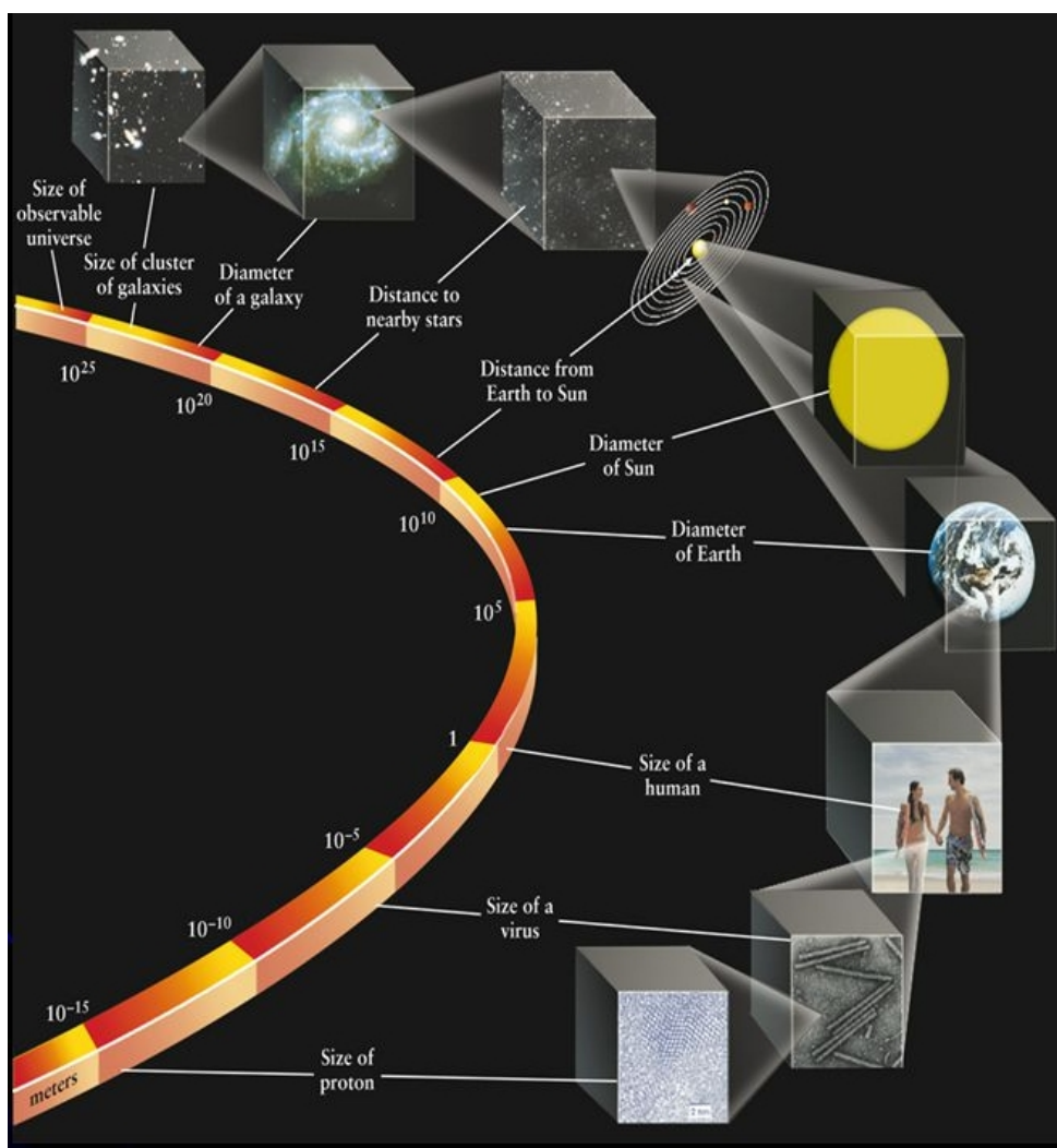
Obrázek 2.5: Velikosti objektů a vzdálenosti ve vesmíru. Převzato z prezentace Neil F. Comins, William J. Kaufmann III, Discovering the Universe .
