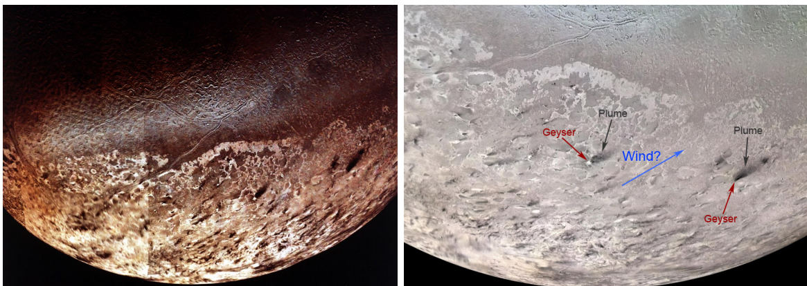
Obrázek 12.31: Vlevo: Povrch největšího Neptunova měsíce – Tritonu. Vpravo: Gejzíry tekutého dusíku poblíž jižního pólu Tritonu. Jak se vyvržený materiál snáší zpět na povrch, naznačuje převládající směr proudění atmosféry. Zdroj: NASA.
