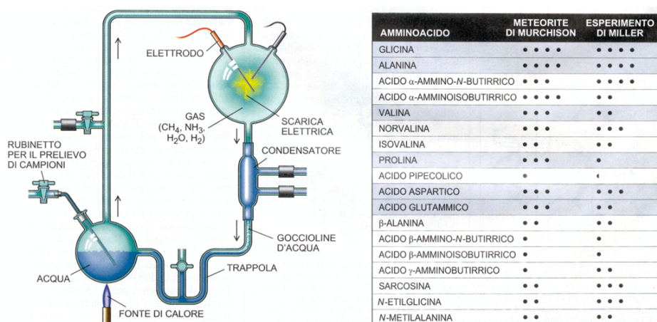
Obrázek 14.2: Aparatura, v níž Miller a Urey simulovali podmínky na Prazemi. V atmosféře z vodíku, metanu a čpavku vznikly s pomocí elektrických výbojů za několik dní značné aminokyseliny a organické sloučeniny (stejně byly objeveny i v Murchinsonském meteoritu). Zdroj: http://www.bionat.unipi.it .
