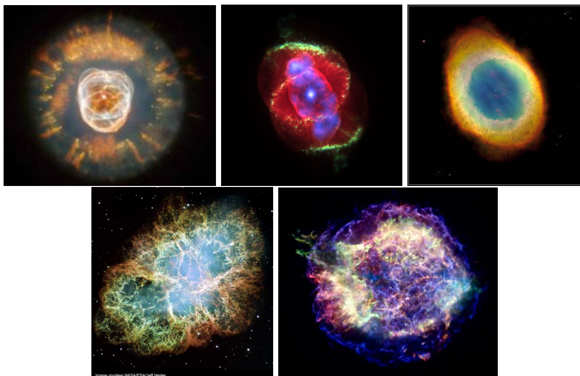
Obrázek 5.13: V horní řadě snímků jsou planetární mlhoviny, zleva Eskymák (NGC 2392), Kočičí oko (NGC 6543) a Prstencová mlhovina (M57) v Lyře a v dolní řadě Krabí mlhovina (M1) v Býku a pozůstatek supernovy v souhvězdí Kasiopeji. Zdroj: Hubble Heritage.
