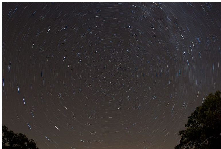
Obrázek 3.3: Hvězdná obloha v okolí severního světového pólu. Znalci hvězdné oblohy jistě neuje Velký vůz nebo hvězdy v souhvězdí Kasiopeja. Převzato z http://planetarium.ipd.org .
