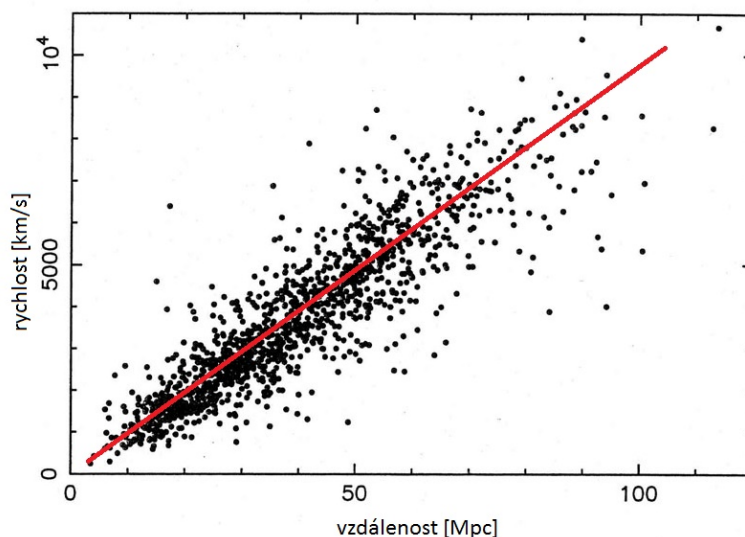
Obrázek 2.8: Závislost rychlosti vzdalování galaxií na jejich vzdálenosti od nás pro 1355 galaxií. Proložená přímka značí Hubbleův zákon. Převzato z Liddle (2005).
