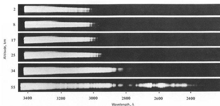
Obrázek 7.11: První fotografie ultrafialového spektra Slunce pořízená z rakety V2 10. října 1946. Tým pod vedením Richarda L. Touseyho ukázal, že s rostoucí výškou nad zemí roste množství zachyceného ultrafialového záření ze Slunce. Zdroj: NASA.
