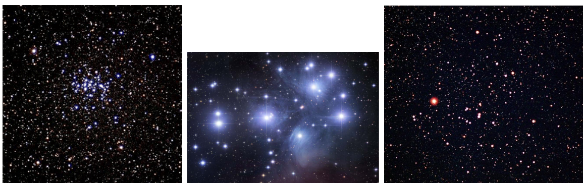
Obrázek 5.10: Otevřené hvězdokupy. Zleva Jesličky (M44), Plejády (M45) a Hyády.
