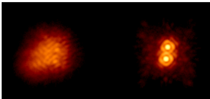
Obrázek 10.18: Dvojhvězda IW Tau pozorovaná pomocí 5m Haleova dalekohledu na Mt. Palomaru. Vlevo: snímek dvojhvězdy bez použití adaptivní optiky; vpravo: odhalené složky dvojhvězdy vzdálené jen 0.3" po využití adaptivní optiky. Převzato z http://www.astro.caltech.edu/palomar/AO/ .
