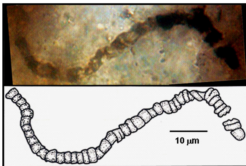
Obrázek 14.1: Mikrofosílie objevené v r. 1992 v Austrálii. Teprve koncem roku 2017 se podařilo využitím nových metod prokázat, že jde o pozůstatky živých organismů. Jejich stáří bylo určeno na 3,5 miliardy let. Zdroj: J. William Schopf, UCLA.
