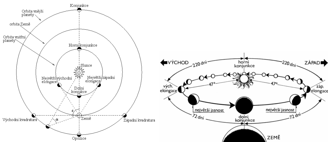
Obrázek 6.26: Aspekty. Zdroj: wikipedia, Příhoda (2000).
