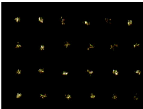
Obrázek 5.16: Vliv astronomického seeingu na kvalitu obrazu hvězdy na snímku. Na obrázku jsou snímky hvězdy pořízené na větším amatérském dalekohledu web kamerou s expoziční dobou 0,01 s. Mezi snímky byla vždy prodleva zhruba jedna sekunda. Převzato z http://www.vikdhillon.staff.shef.ac.uk/ .
