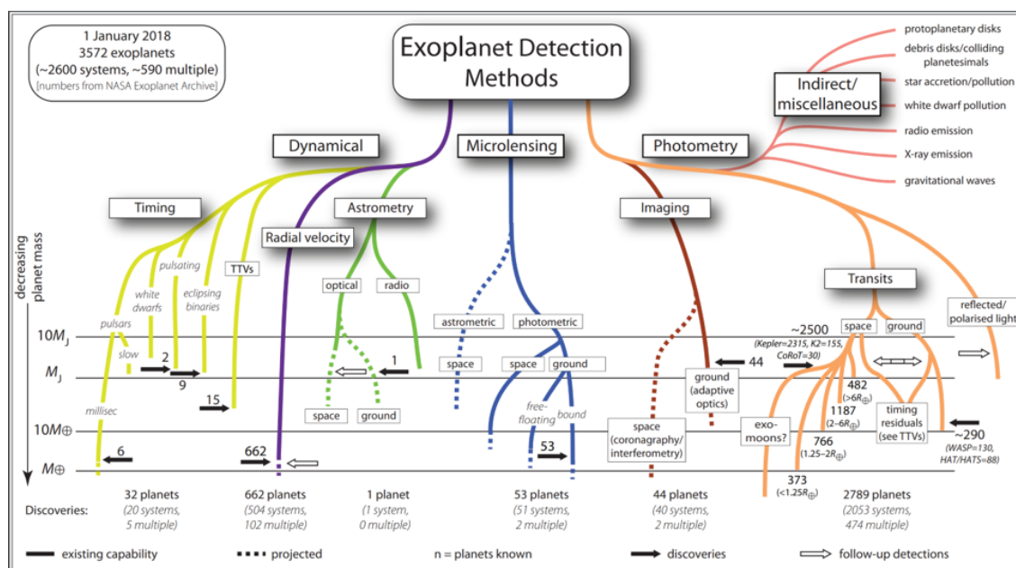
Obrázek 13.3: Perrymanův diagram metod detekce exoplanet. Stav k 1. 1. 2018. Převzato z ExoverseTeamReport.pdf
