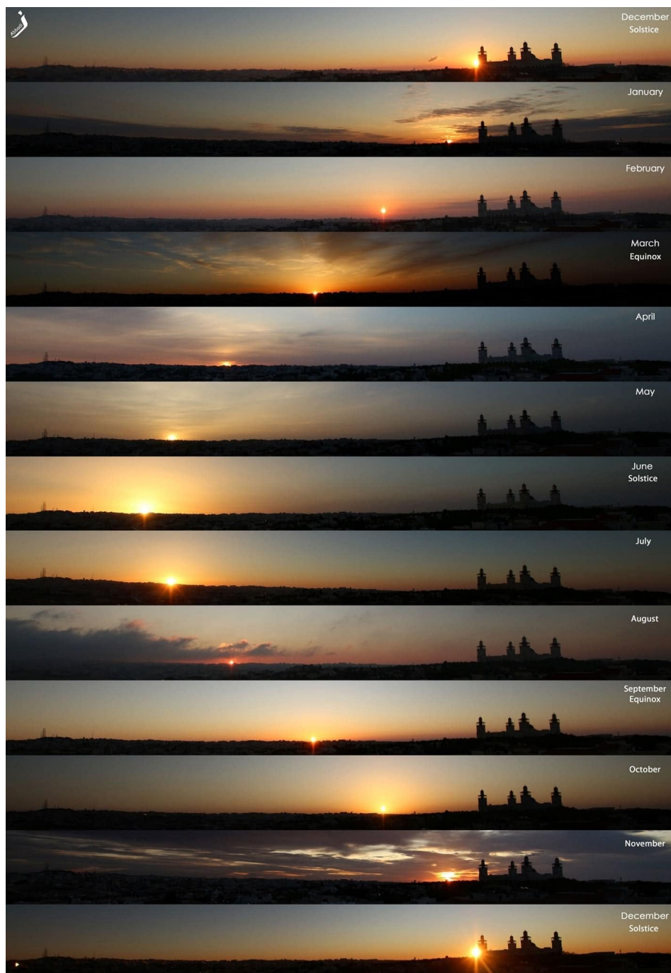
Obrázek 6.2: Východy Slunce v Ammánu (Jordánsko) v průběhu roku 2019; https://apod.nasa.gov/apod/ap201221.html . Foto: Zaid M. Al-Abbadi.
