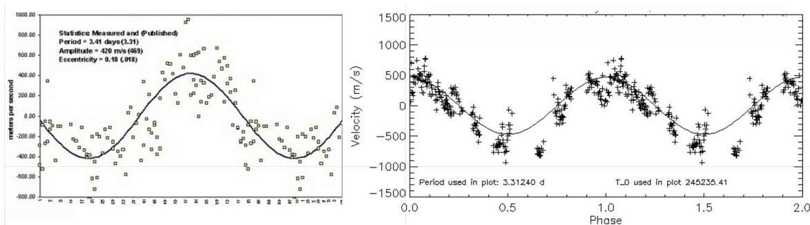
Obrázek 13.9: Křivka radiálních rychlostí hvězdy \tau Boo jasně ukazuje přítomnost exoplanety. Měření byla provedena skupinou amatérských astronomů v letech 2000 (obrázek vlevo) a 2004. Převzato z http://www.spectrashift.com .
