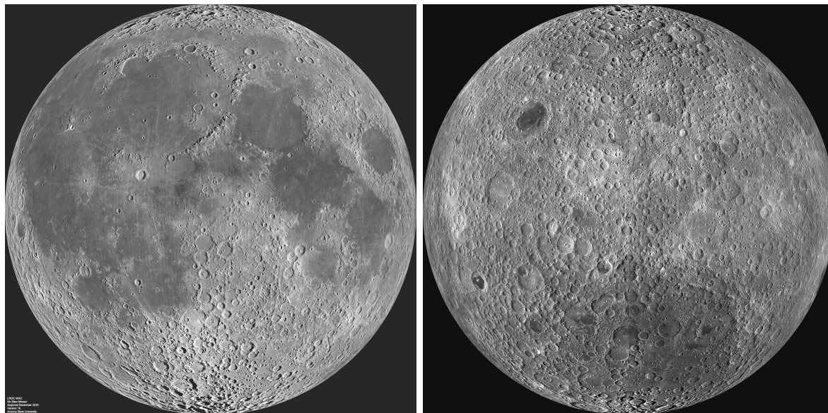
Obrázek 6.10: Přivrácená a odvrácená strana Měsíce ze sondy Lunar Reconnaissance Orbiter. Zdroj: NASA.
