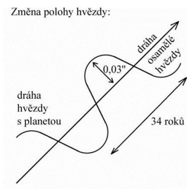
Obrázek 13.5: Možnosti astrometrické detekce exoplanet. Převzato z Pokorný (2006).
