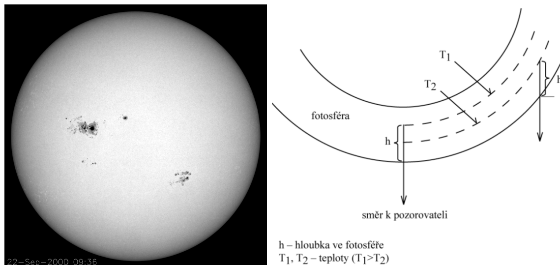
Obrázek 7.19: Vlevo: Okrajové ztemnění je u našeho Slunce jasně patrné. Snímek převzat z http://sohowww.nascom.nasa.gov/hotshots/2000.09.22/ . Vpravo: Schématické znázornění vzniku okrajového ztemnění. Převzato z Pokorný (2006).
