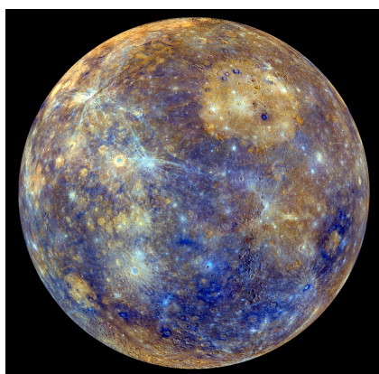
Obrázek 12.5: Snímek Merkuru z širokoúhlé kamery sondy Messenger. Zdroj: NASA.
