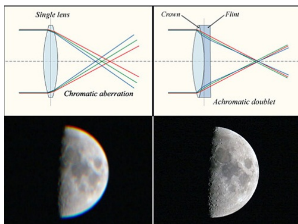
Obrázek 10.15: Levný dalekohled s jednoduchou čočkou vytváří rozmazaný obraz s okrají s falešnými barvami (vlevo). Galileoscope (vpravo) představuje kvalitnější achromát tvořený dvojitou čočkou. Ohnisko je společné pro modré a červené světlo, ohnisko zeleného světla je lehce posunuté. Zdroje: Schémata R. Caniatti/Wikipedia, snímky Měsíce R. Fienberg.
