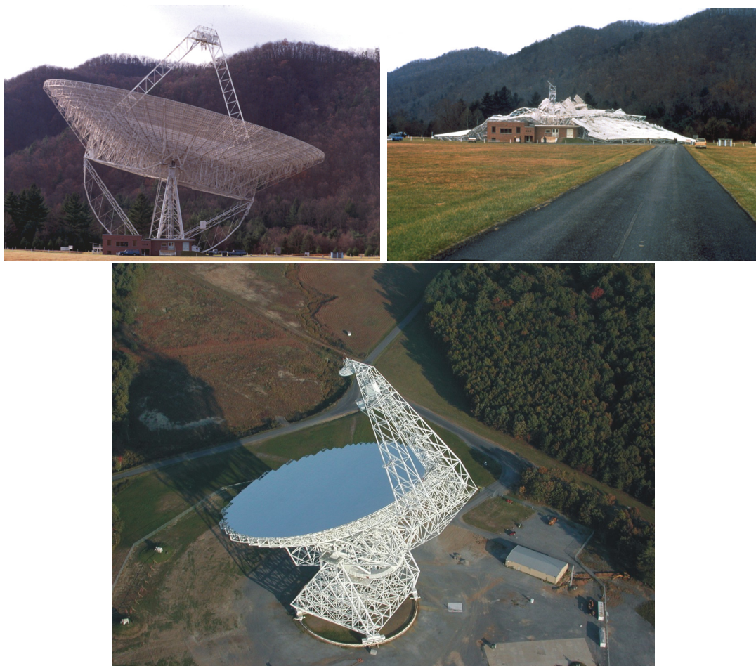
Obrázek 11.4: Nahoře: Původní velký radioteleskop v NRAO, Green Bank, 15. listopadu 1988 a vpravo následující den, po zhroutil. Dole: Zničený radioteleskop nahradil nový přístroj – Robert C. Byrd Green Bank Telescope. Foto: Richard Porcas, NRAO.
