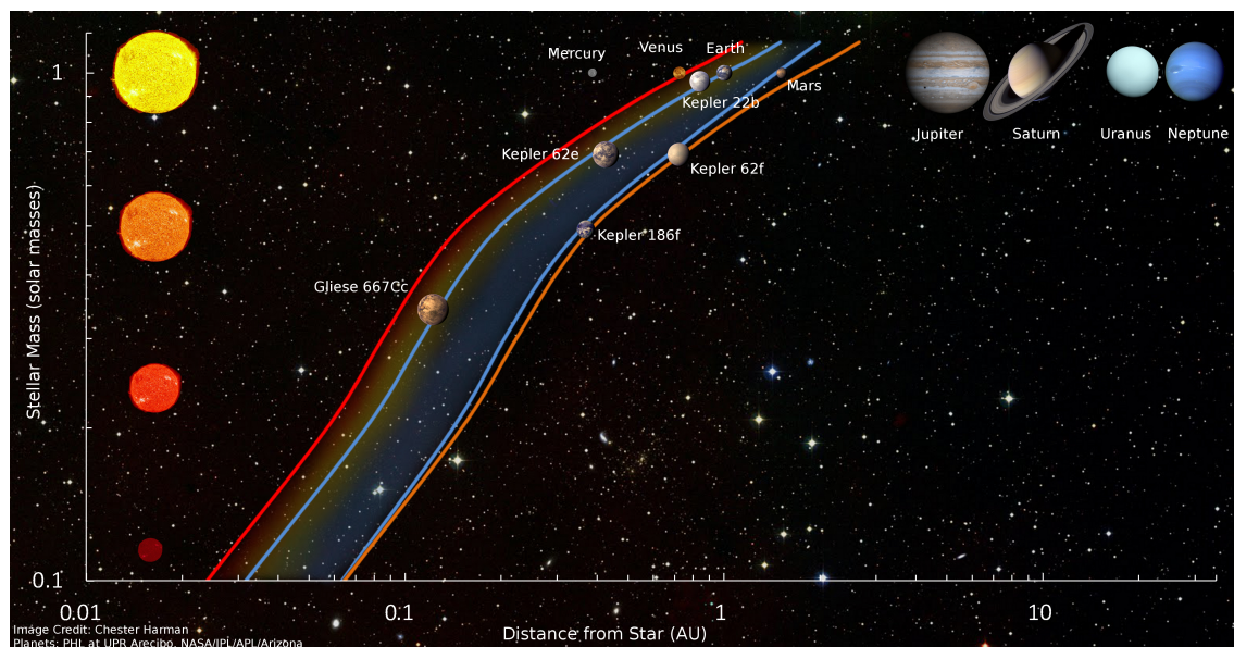
Obrázek 14.4: Zóny života u různých typů hvězd. Jejich vzdálenost od mateřské hvězdy a rozsah je ovlivněn její povrchovou teplotou. Autor: S. Harman, NASA/JPL/APL/Arizona.
