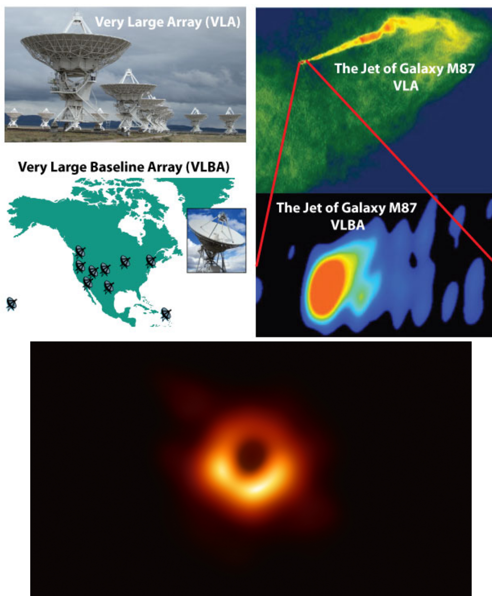
Obrázek 11.6: Nahoře vlevo: radioteleskopy použité v interferometrické soustavě VLA, respektive VLBA. Nahoře vpravo: porovnání výsledků při pozorování výtrysku z galaxie M87. Zdroj: http://www.erau.edu/ . Dole: První snímek černé díry v centru galaxie M87 pořízený EHT. Zdroj: ESO.
