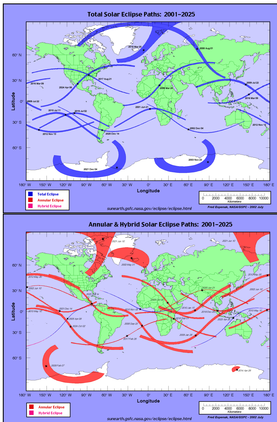
Obrázek 6.20: Pásy, odkud jsou pozorovatelná úplná, prstencová a hybridní zatmění Slunce. Zdroj: F. Espenak, NASA.
