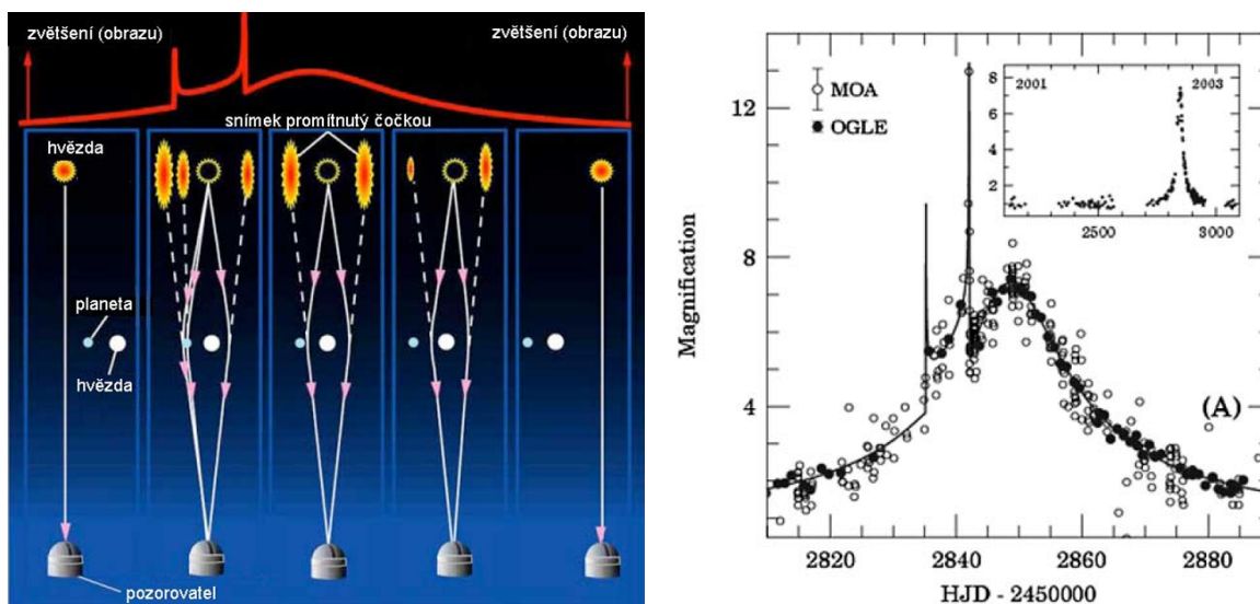
Obrázek 13.6: Vlevo: Ilustrace metody gravitační mikročocky v detekci exoplanet. Převzato z http://astronomia.zcu.cz . Vpravo: Pozorování planety gravitační mikročockou v projektu OGLE (Bond et al., 2004). Vložený obrázek ukazuje všechna měření hvězdy z projektu OGLE v letech 2001 až 2003. Hlavní obrázek ukazuje bližší pohled na data z roku 2003 ze dvou projektů OGLE a MOA.
