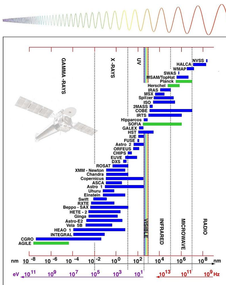
Obrázek 10.22: Významné astronomické observatoře v kosmu do r. 2005. Zdroj: https://www.wikiwand.com
