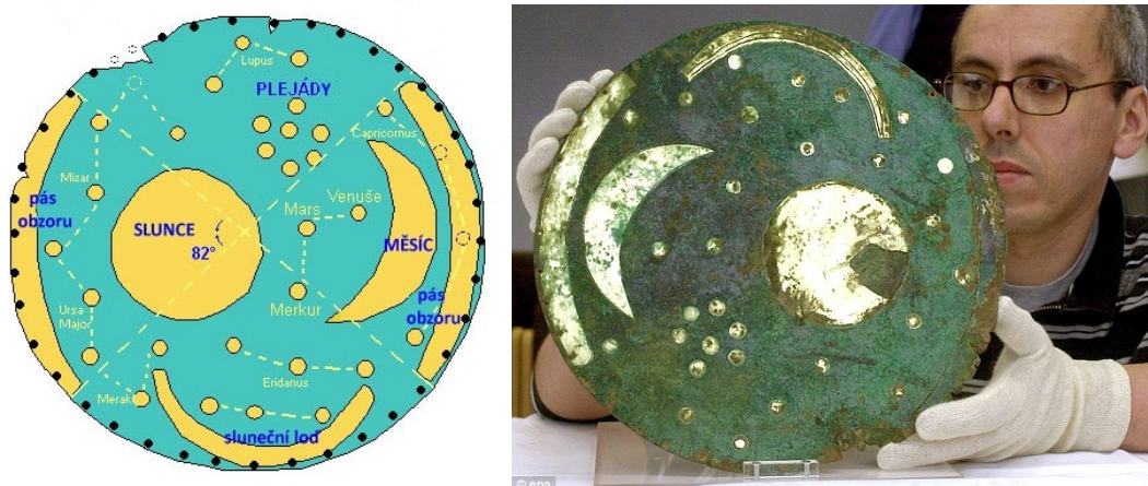
Obrázek 1.4: Disk z Nebry. Upomínka na astronomii doby bronzové. Byl vyroben mezi roky 2100 až 1700 př.n.l. a později několikrát upravován. Jde o jedno z nejstarších vyobrazení oblohy s astronomickými objekty. Památka UNESCO v programu Paměť světa. Zdroje: http://www.celticnz.co.nz/NebraSunDisk/NebraSunDisk.htm (schéma; upraveno), http://www.dailymail.co.uk/ .
