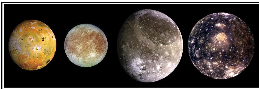
Obrázek 12.28: Galileovské družice Io, Ganymed, Europa, Kallisto. Zdroj: NASA.
