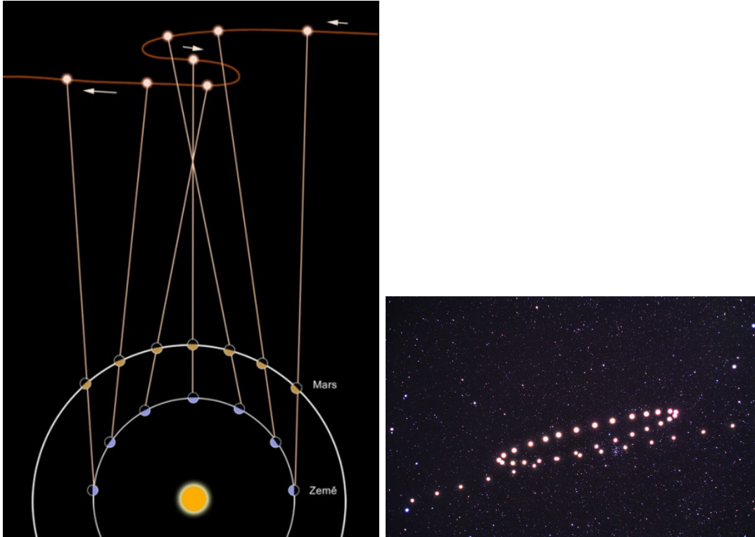
Obrázek 6.25: Vlevo: schematický náčrt vzniku smyček planet na hvězdné obloze. Převzato z Astronomického koutku. Autor: Ota Kéhar. Vpravo: Smyčka planety Mars v souhvězdí Raka v období říjen 2009 až květen 2010. Foto Tunc Tezel.
