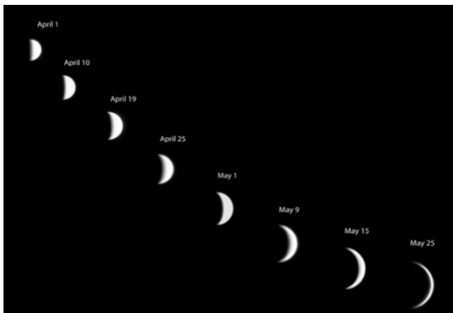
Obrázek 6.22: Fáze Venuše v dubnu a květnu 2004. Foto: John Rummel.
