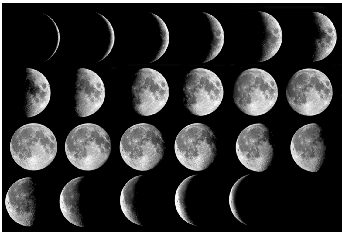
Obrázek 6.8: Fáze Měsíce. Foto: A. Cidadao.
