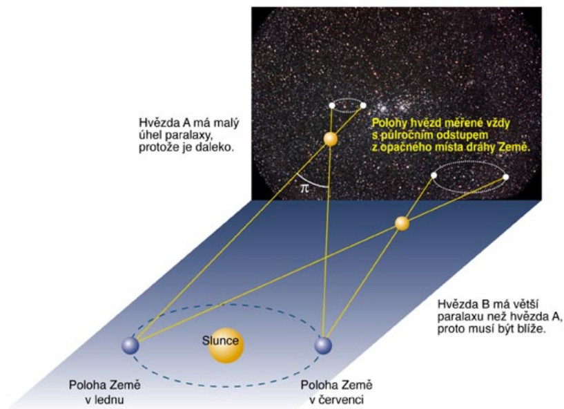
Obrázek 2.7: Trigonometrická metoda pro určování vzdálenosti hvězd. Zdroj: http://hvezdy.astro.cz .
