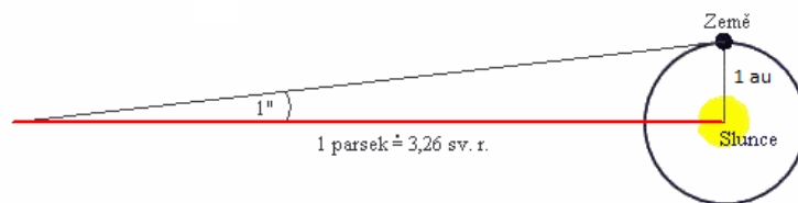
Obrázek 2.4: K definici parseku. Zdroj: http://hvezdy.astro.cz .
