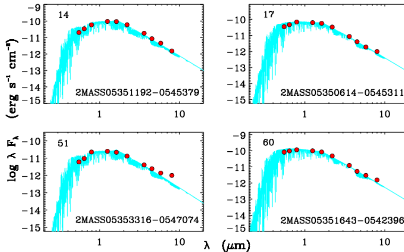
Obrázek 9.3: Rozložení energie ve spektru (SED; Spectral energy distribution) čtyř hvězd z katalogu 2MASS. Červené body představují výsledky fotometrických měření, světle modře je zobrazen uměle spočtené spektrum hvězd, které nejlépe odpovídá fotometrickým pozorováním. Zdroj: Frasca et al. (2009).
