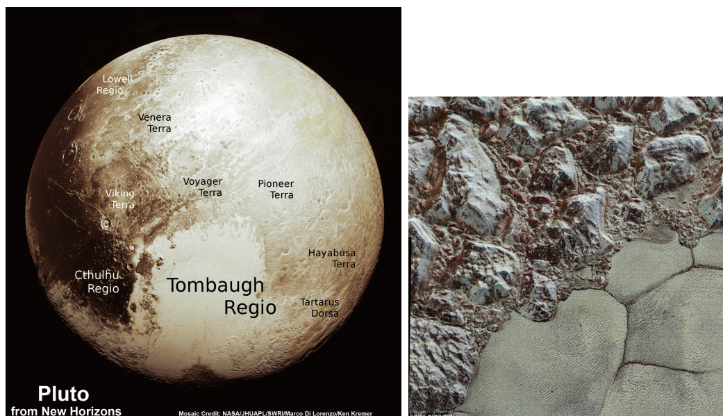
Obrázek 12.24: Vlevo: Nový celkový pohled na Pluto vytvořený ze snímků sondy New Horizons pořízených 14. 7. 2015 ze vzdálenosti 80 000 km od povrchu. Vpravo: Detailní snímek planiny Sputnik na povrchu Pluta. Zdroj: NASA.
