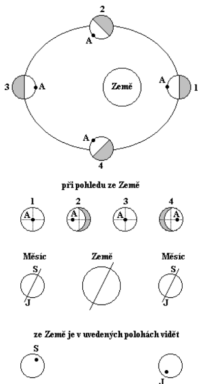
Obrázek 6.12: Vlevo: Schématické znázornění librace Měsíce. Zdroj: http://fyzika.jreichl.com/main.article/view/1008-rotace-mesice . Vpravo nahoře: librace v délce, dobře patrná podle červeného bodu v Moři nepokojů. Zdroj: Steve Schimmrich. Vpravo dole: librace v šířce. Výborným orientačním bodem je kráter Tycho. Zdroj: John Chumack (vlevo), Frank Barrett (vpravo).
