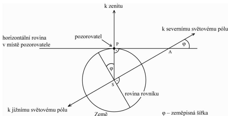
Obrázek 3.4: Odvození závislosti úhlové výšky Polárky na zeměpisné šířce pozorovacího stanoviště.
