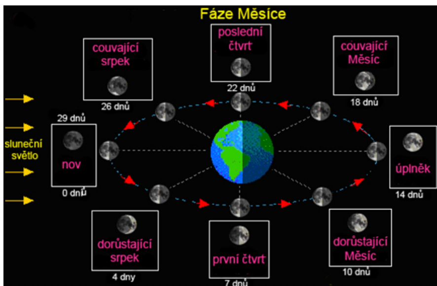
Obrázek 6.7: Vznik fází Měsíce. Zdroj: http://leccos.com .
