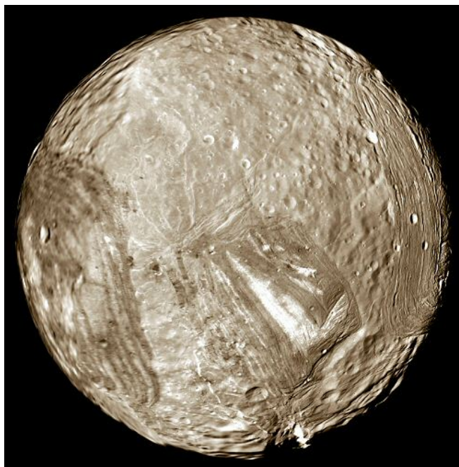
Obrázek 12.30: Uranova družice Miranda na snímku pořízeném sondou Voyager 2 v roce 1986. Zdroj: NASA.
