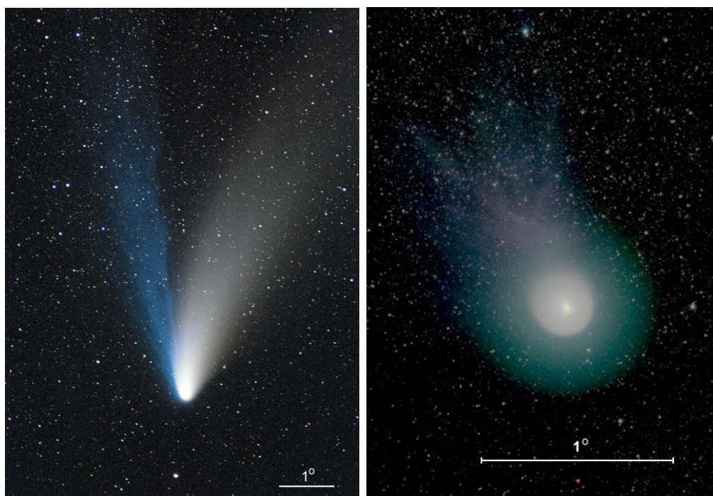
Obrázek 6.27: Vlevo: Kometa Hale-Bopp s modrým plynovým a nažloutlým prašným ohonem. Foto: Miloslav Druckmüller, 2. 4. 1997. Vpravo: Kometa 17P/Holmes s obří komou. Foto: AnnMarie Jones (5. 11. 2007).
