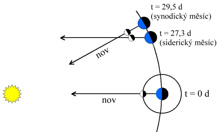
Obrázek 6.6: Synodický a siderický měsíc. Zdroj: http://www.astronomy.ohio-state.edu/ .
