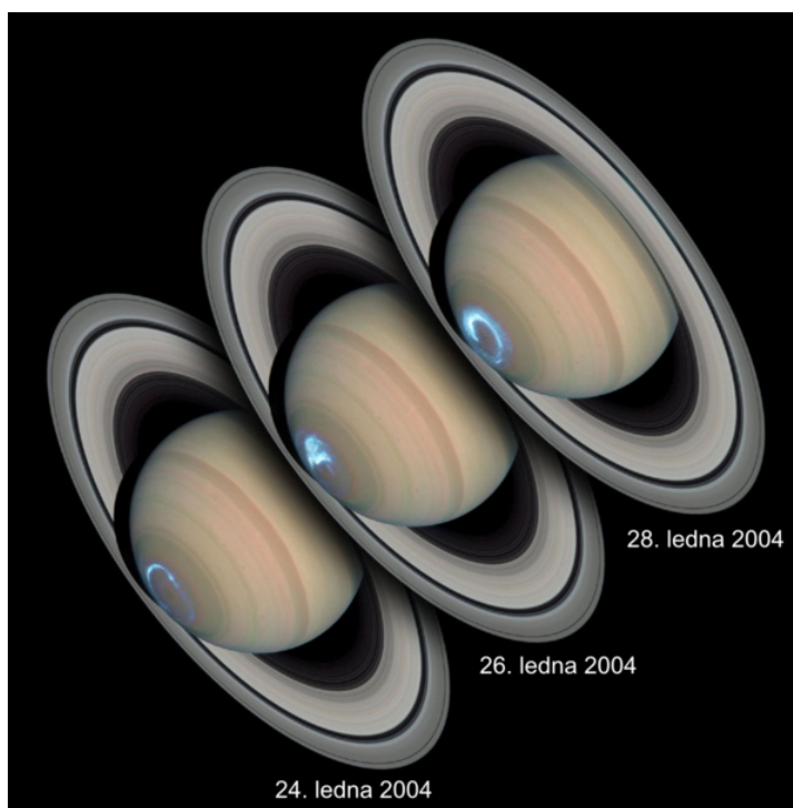
Obrázek 12.18: Polární záře na Saturnu. Trojice snímků vznikla kombinací snímků v ultrafialovém a viditelném spektru, přičemž ultrafialové záběry vznikly v lednu 2004 za pomoci Hubbleova vesmírného dalekohledu a snímky ve viditelné oblasti spektra až v březnu téhož roku. Zdroj: NASA, ESA.
