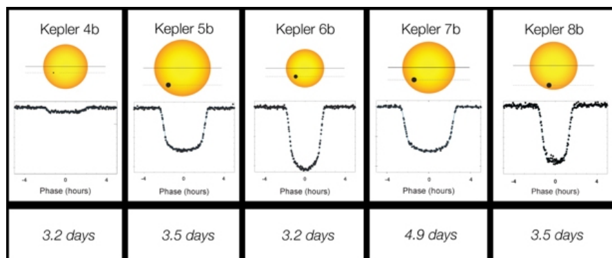
Obrázek 13.11: Ukázka tranzitů pěti exoplanet pozorovaných družicí KEPLER. Zdroj: NASA.
