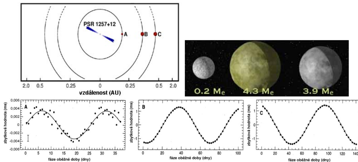
Obrázek 13.8: Nahoře: Pulsar PSR 1257+12 a jeho planetární soustava. Dole: Zbytkové hodnoty času z měření pulsaru PSR 1257+12, na kterých je vidět vliv oběžných dob 25,34 dne (planeta A; dle později přijatých pravidel planeta b pojmenovaná Draugr), 66,54 dne (planeta B; c, Poltergeist) a 98,22 dne (planeta C; d, Phobetor). Pozorování bylo prováděno po dobu 3 let. Na každém snímku je vliv ostatních dvou planet odfiltrován. Pro planetu A je na snímku zřetelná nejistota výsledku, která je důsledkem digitálního zpracování signálu. Pro planety B a C jsou nejistoty nepostřehnutelné. Převzato z http://astronomia.zcu.cz .
