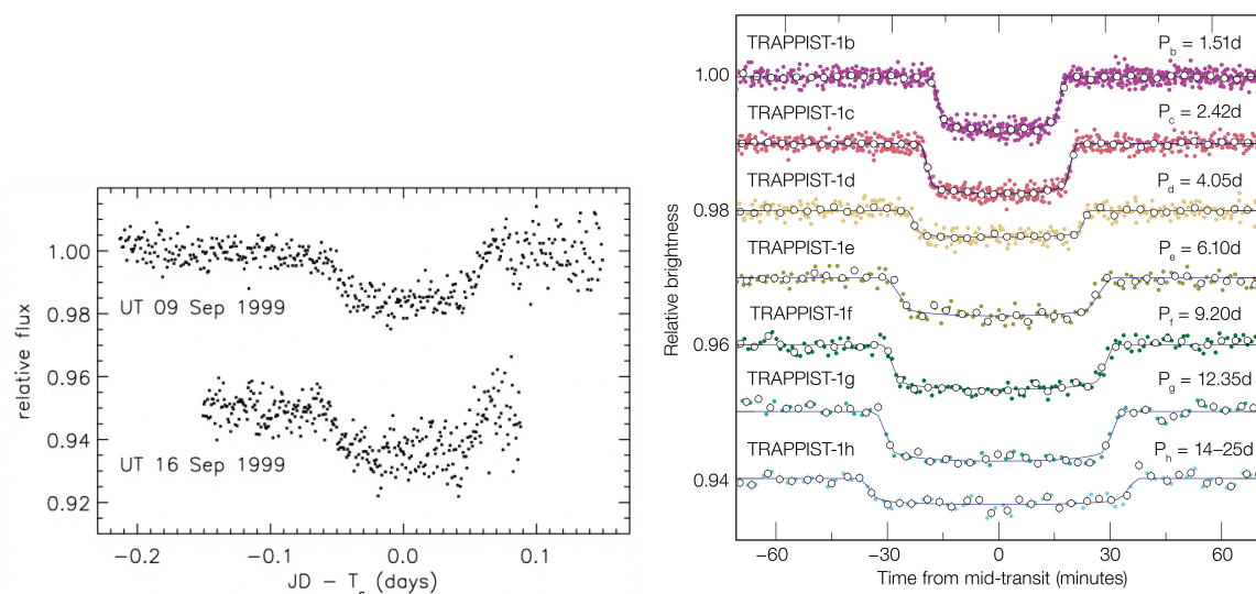
Obrázek 13.10: Vlevo: První zaznamenané tranzity exoplanety HD 209458 b. Zdroj: Charbonneau et al. (2000). Vpravo: Transit planet v unikátní soustavě TRAPPIST-1. Zdroj: https://www.eso.org/public/news/eso1706/
