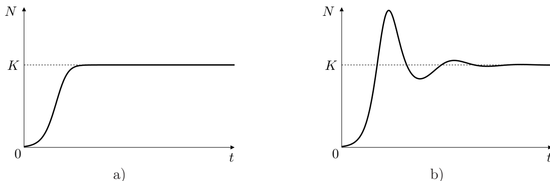
Obrázek 7.2: Průběh řešení úlohy (7.3), (7.5). a) \delta = 4r , b) \delta = \frac{1}{2}r .
