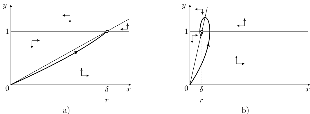
Obrázek 7.1: Fázový portrét systému (7.4) a jeho trajektorie s počáteční podmínkou 0 < x(0) \ll 1 , y(0) = 0 . a) \delta \geq 4r , b) \delta < 4r . Oba obrázky mají stejné měřítko na ose x .
