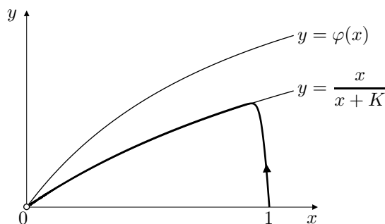
Obrázek 8.3: Nulklina systému (8.9) a jeho trajektorie s počáteční podmínkou (8.10) a hodnotou parametru \varepsilon = \frac{1}{10} .
