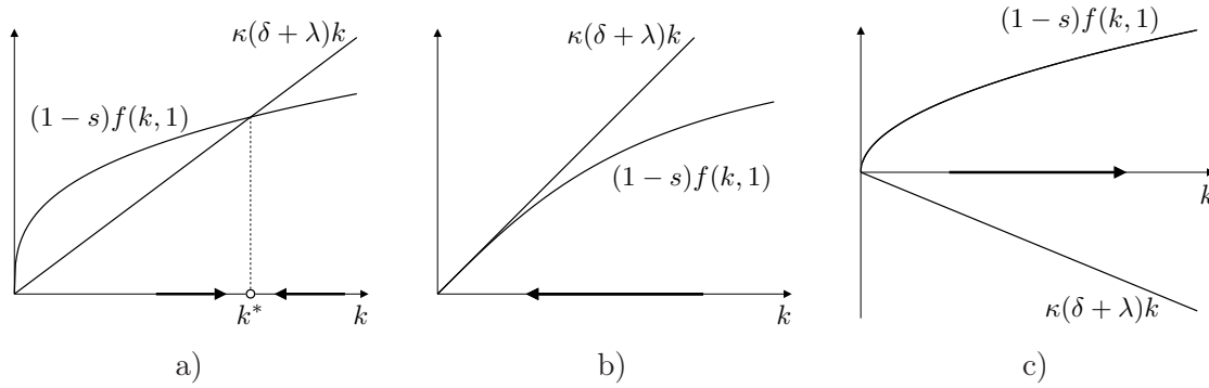
Obrázek 9.1: Řešení rovnice (9.14) pro stacionární bod k^* základní dynamické rovnice neoklasického modelu (9.13). Na vodorovné ose je současně fázový portrét rovnice (9.13). a) \delta + \lambda > 0 a je splněna podmínka (9.15). b) Není splněna podmínka (9.15). c) Neplatí \delta + \lambda > 0 .
