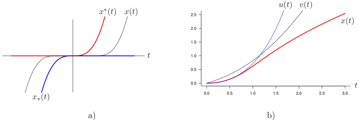
Obrázek 2.3: a) Maximální a minimální řešení počáteční úlohy (2.19). b) Odhady řešení x = x(t) úlohy (2.20) s hodnotami t_0 = x_0 = 0 .
