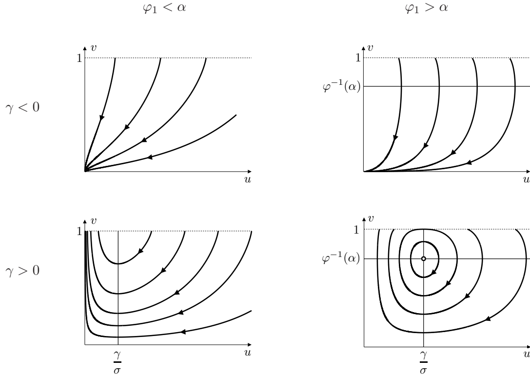
Obrázek 9.2: Trajektorie a nulklíny systému (9.36) pro možné kombinace parametrů
