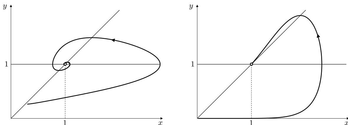
Obrázek 4.4: Trajektorie systému (4.12) se dvěma různými hodnotami parametru \varrho . Vlevo: \varrho = 0,5 a stacionární bod je ohnisko, vpravo: \varrho = 8 a stacionární bod je uzel.
