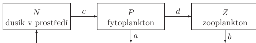
Obrázek 6.1: Schéma koloběhu dusíku
