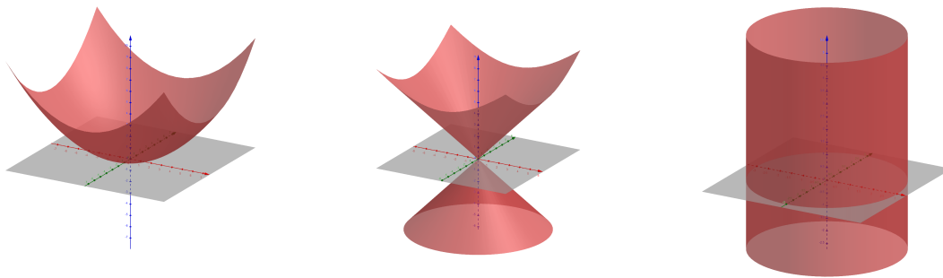
Obrázek 26.3: Rotační paraboloid, rotační kuželová a rotační válcová plocha
