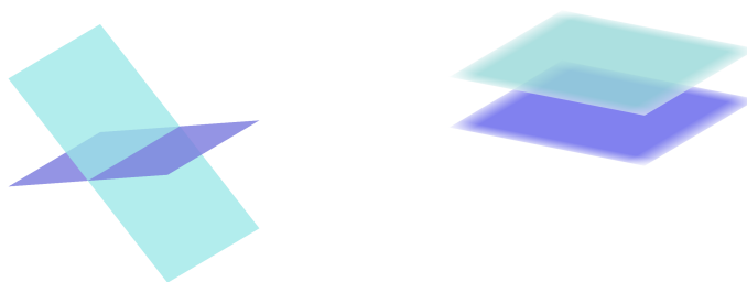
Obrázek 24.12: Různoběžné a rovnoběžné roviny
