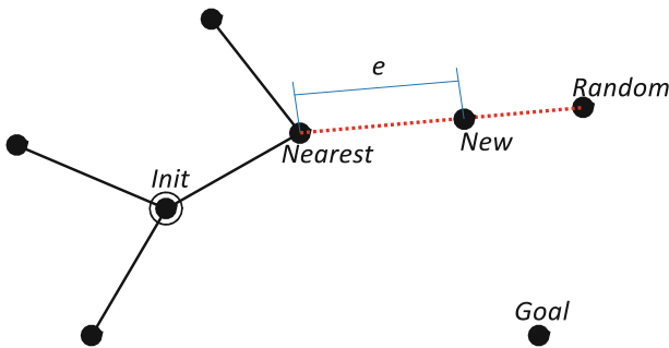
Fig. 1. RRT principle
