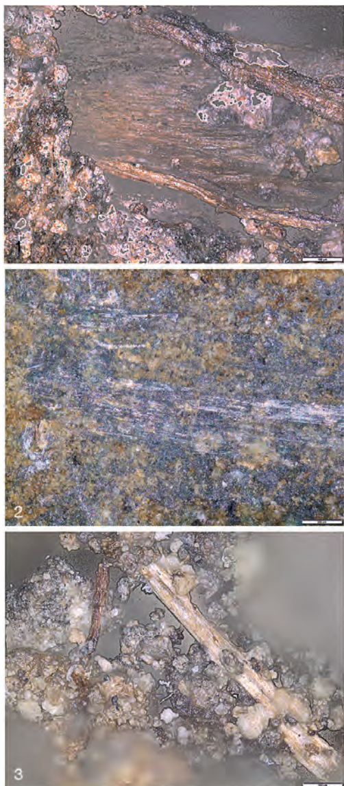
Obr. 14. 1 – mikrorezidua dřeva v sedimentu odebraném z bronzové břitvy, zvětšení 200x; 2 – stopy broušení na příčném ostří bronzové břitvy, zvětšení 100x; 3 – hustě uložená mikrorezidua dřeva, dochovaná ve svazcích a větších plochách v záhlaví čepele bronzové dýky, zvětšení 200x.
