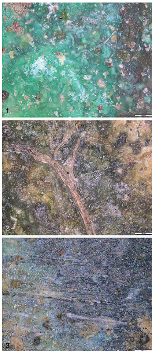
Obr. 15. 1 – mikrorezidua textilních vláken pohřbená v patině čepele bronzové dýky, zvětšení 200x; 2 – mikrorezidua textilních vláken promísená s mikrorezidui dřeva na čepeli bronzové dýky, zvětšení 200x; 3 – stopy broušení na čepeli bronzové dýky, zvětšení 200x.
