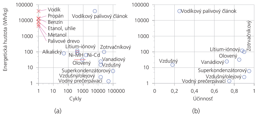
Obrázok 26.13 Niektoré vlastnosti systémov uskladňovania a palív. (a) Energetická hustota (na logaritmickej mierke) oproti životnosti (počet cyklov). (b) Energetická hustota oproti účinnosti. Energetické účinnosti nezahŕňajú hmotnosti nádrží energetických systémov, okrem „vzduchu“ (uskladňovanie stlačeným vzduchom). Ak zoberieme do úvahy váhu kryogenickej nádrže pre uskladňovanie vodíka, jeho energetická hustota klesá z 39 000 Wh/kg na zhruba 2 400 Wh/kg.
