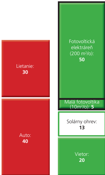
Obrázok 6.9 Fotovoltaika: 10 m 2 článkov na každom dome na južne orientovaných strechách s 20 % účinnosťou dokáže dodávať 5 kWh elektrickej energie za deň. Ak by sa pokrylo 5 % krajiny článkami s 10 % účinnosťou (200 m 2 článkov na osobu), mohli by dodať 50 kWh/deň/osobu.
