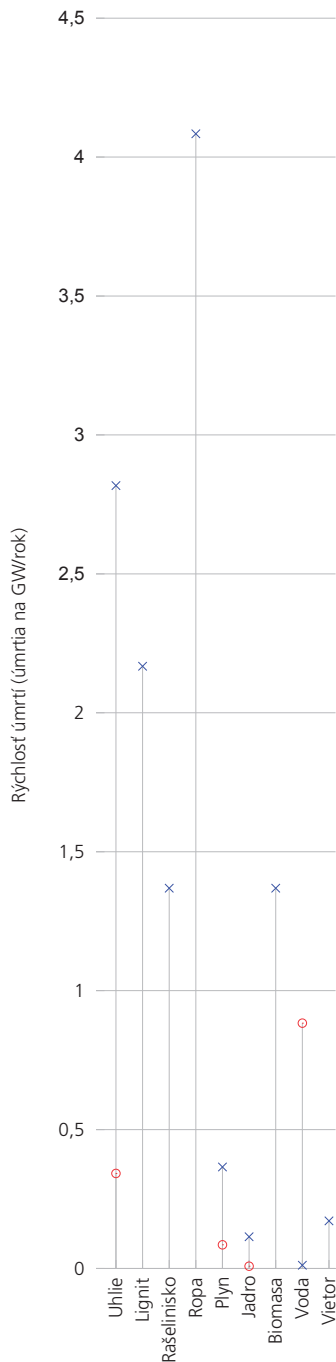
Obrázok 24.11 Úmrtnosť v závislosti od použitej technológie produkcie elektriny. x: odhady v rámci EÚ podľa projektu ExternE. o: podľa Inštitútu Paula Scherrera.
